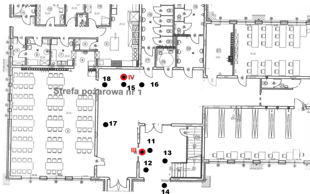
Rys. 1b: Plan rozmieszczenia punktów pomiarowych – parter część 2 (dawne Gimnazjum) kolorem czerwonym oznaczono lokalizację punktów dostępnych
