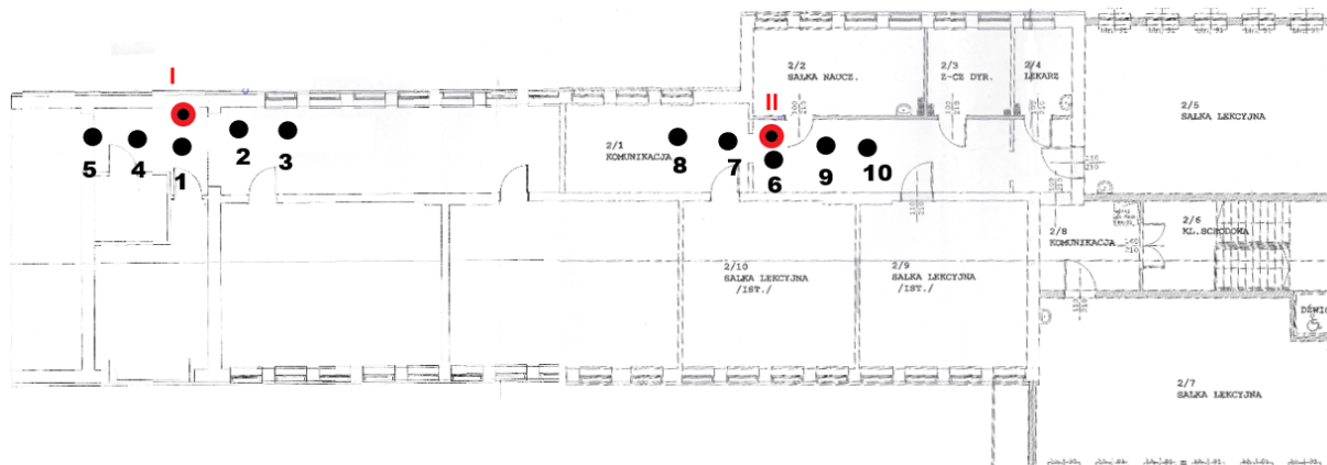
Rys. 1a: Plan rozmieszczenia punktów pomiarowych – parter część 1 kolorem czerwonym oznaczono lokalizację punktów dostępnych
