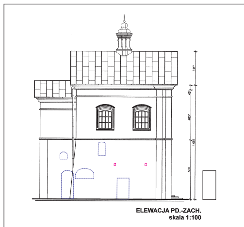
4. Leśna Podlaska – zespół klasztorny oo. Paulinów, kaplica Zjawienia, elewacja pd. z wynikami badań architektonicznych, oprac. J. Maraśkiewicz, 2014.
