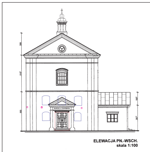
3. Leśna Podlaska – zespół klasztorny oo. Paulinów, kaplica Zjawienia, elewacja wsch. z wynikami badań architektonicznych, oprac. J. Maraśkiewicz, 2014.
