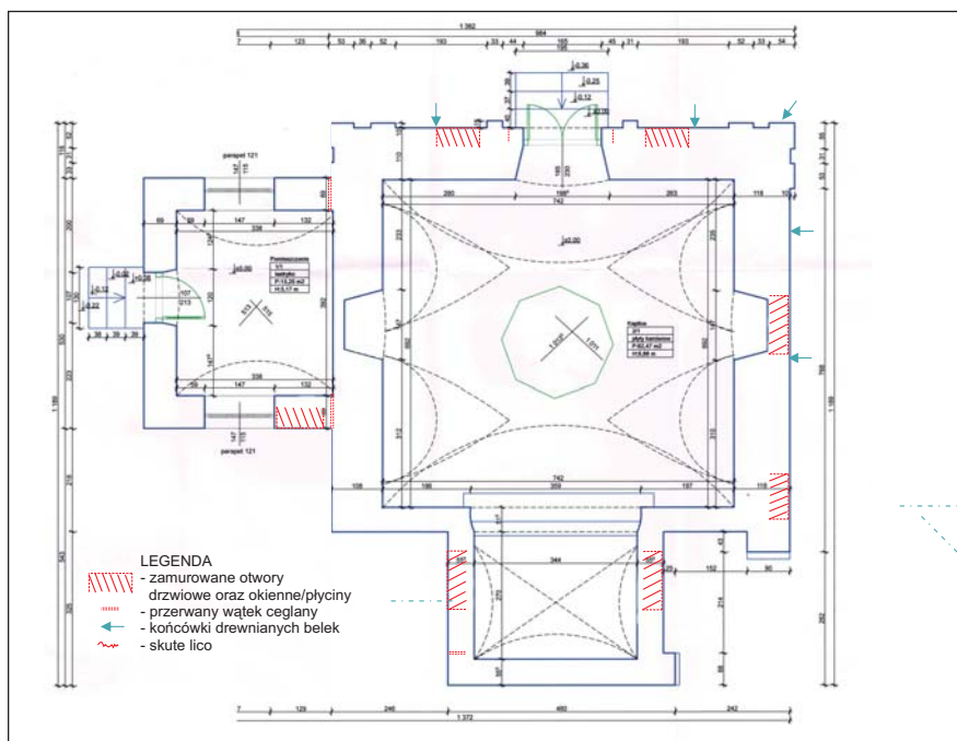
2. Leśna Podlaska – zespół klasztorny oo. Paulinów, kaplica Zjawienia, rzut z wynikami badań architektonicznych, oprac. J. Maraśkiewicz, 2014.
