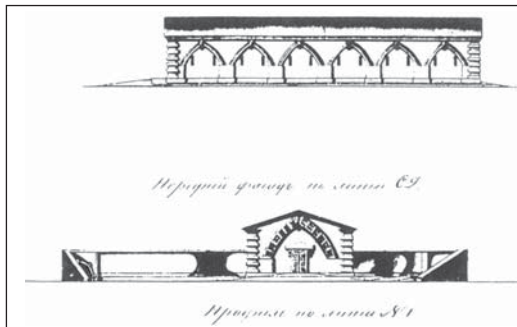
Rys. 1. Zamość, Prochownia, plan budynku oznaczony literą L, 1845 r., oryg. CGWIA Moskwa sygn.F349 op.12d 7132, arch.WUOZ Del. Zamość.
