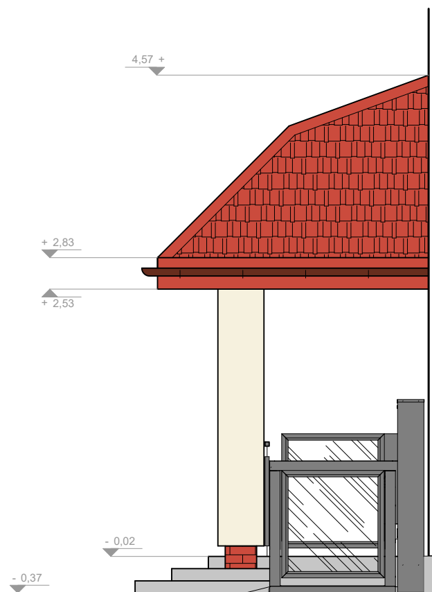
Widok strony prawej
