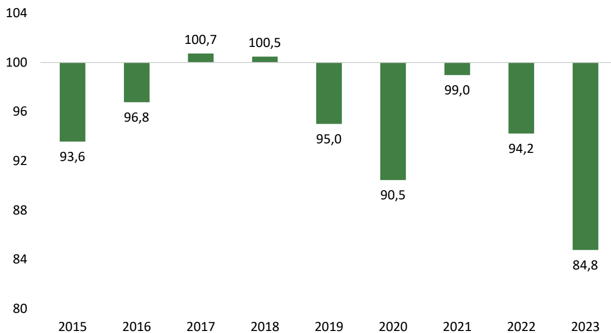
Dynamika emisji CO 2 (2010=100)
