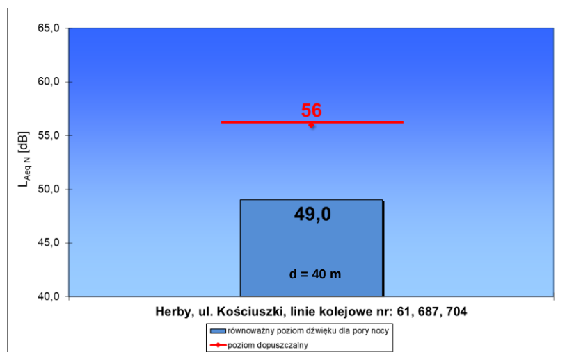
Ryc. 3. Wartość wskaźnika L_{Aeq N} dla rozpatrywanego punktu pomiarowego oraz jego porównanie z obowiązującą wartością poziomu dopuszczalnego, Herby, 2024 rok.
