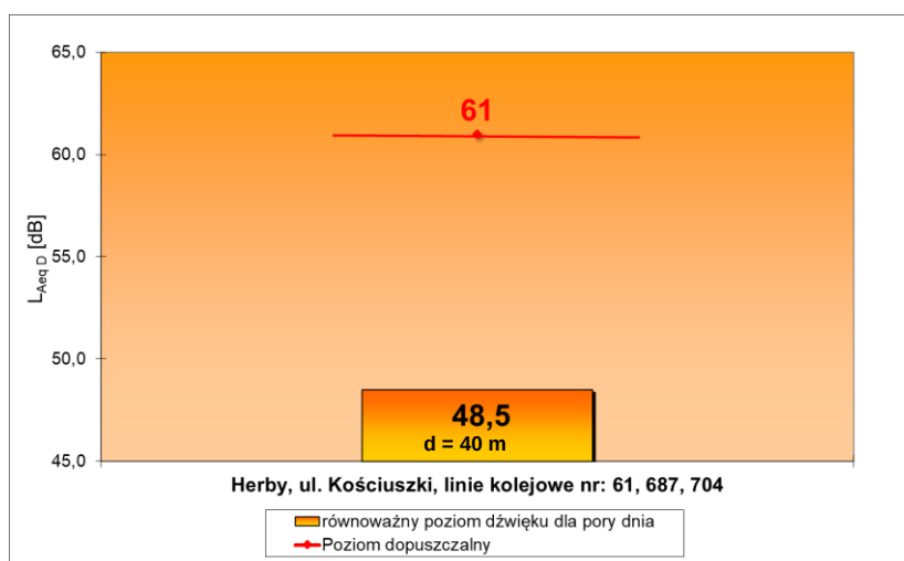
Ryc. 2. Wartość wskaźnika L_{Aeq D} dla rozpatrywanego punktu pomiarowego oraz jego porównanie z obowiązującą wartością poziomu dopuszczalnego, Herby, 2024 rok.
