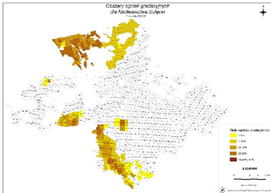
Rys. 2 – Obszary ognisk gradacyjnych na terenie Nadleśnictwa Sulęcín.
