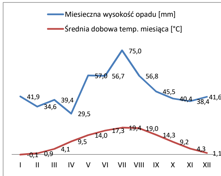
Rysunek 2 Wskaźniki klimatologiczne dla stacji meteorologicznej w Gorzowie Wlkp, w okresie (1991-2020)
