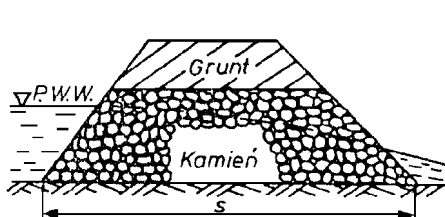
Rys. 1.1. Drogowy nasyp filtracyjny
