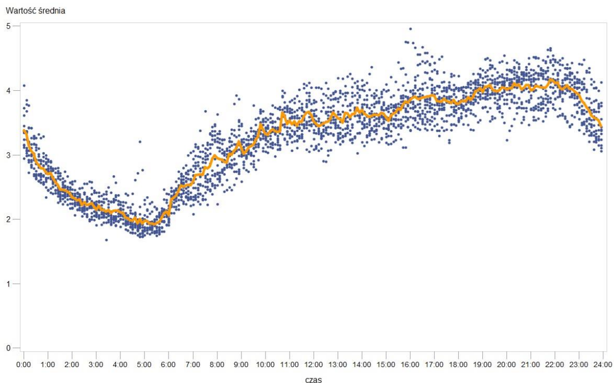
Rys. 7 Wyniki pomiarów – Zakład Wodociągów i Kanalizacji w Szczecinie – średnia za okres 24 godzin
