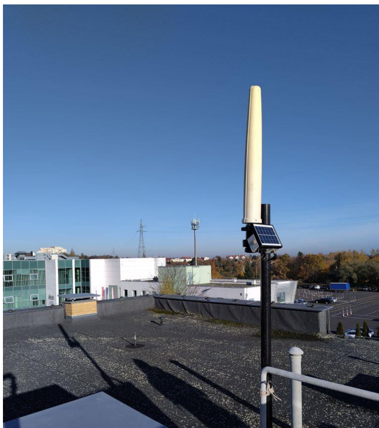
Rys. 2. Miejsce montażu SMS PEM – Zakład Wodociągów i Kanalizacji w Szczecinie
