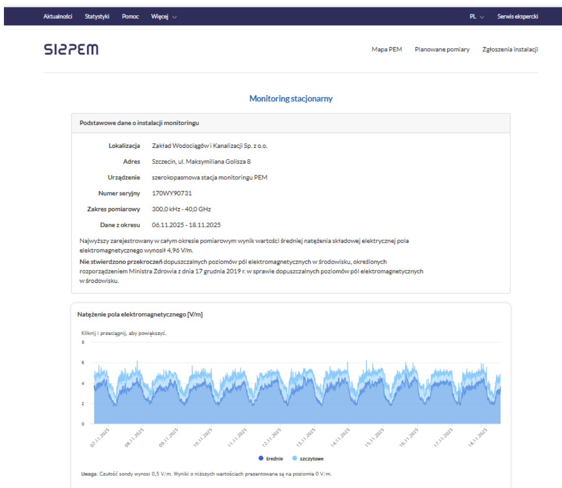
Rys. 17 Obrazowanie wyników monitoringu stacjonarnego PEM – okienko ze szczegółami
