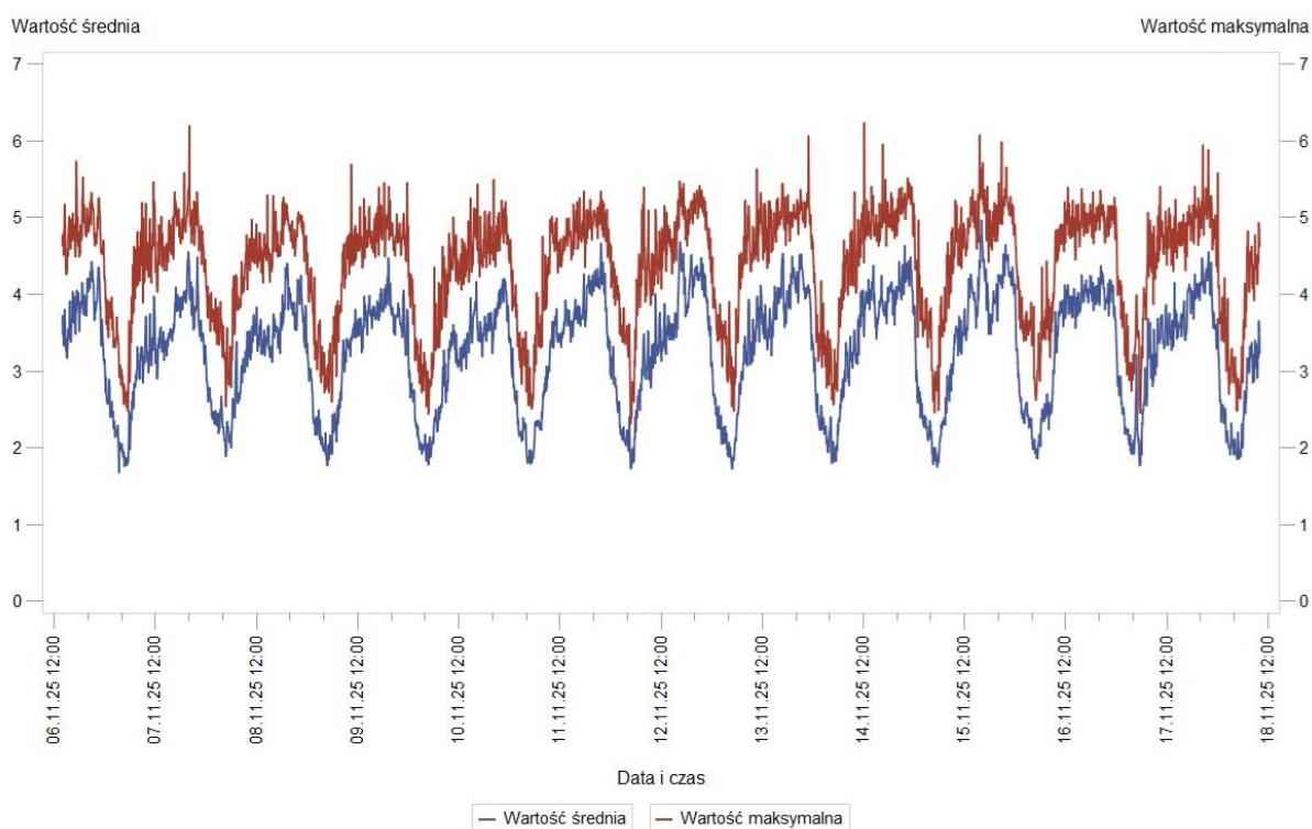
Rys. 6 Wyniki pomiarów – Zakład Wodociągów i Kanalizacji w Szczecinie w dniach 6.11.2025 r. – 18.11.2025 r. – wartość średnia i wartość maksymalna
