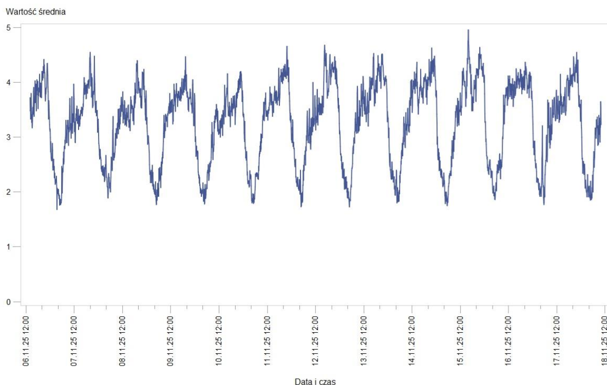
Rys. 5 Wyniki pomiarów – Zakład Wodociągów i Kanalizacji w Szczecinie w dniach 6.11.2025 r. – 18.11.2025 r. – wartość średnia
