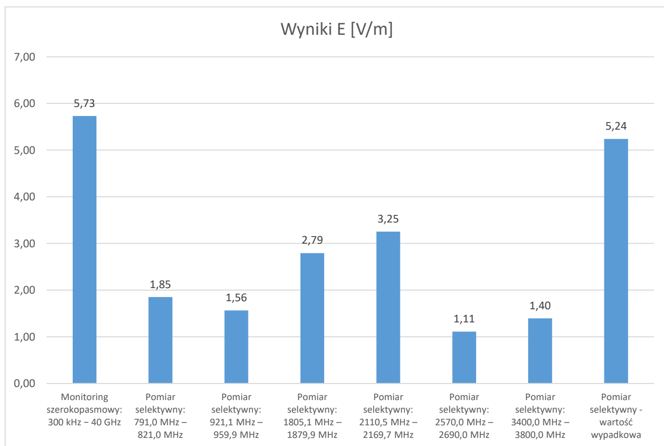
Rys. 15 Porównanie wyników monitoringu szerokopasmowego i pomiarów selektywnych
