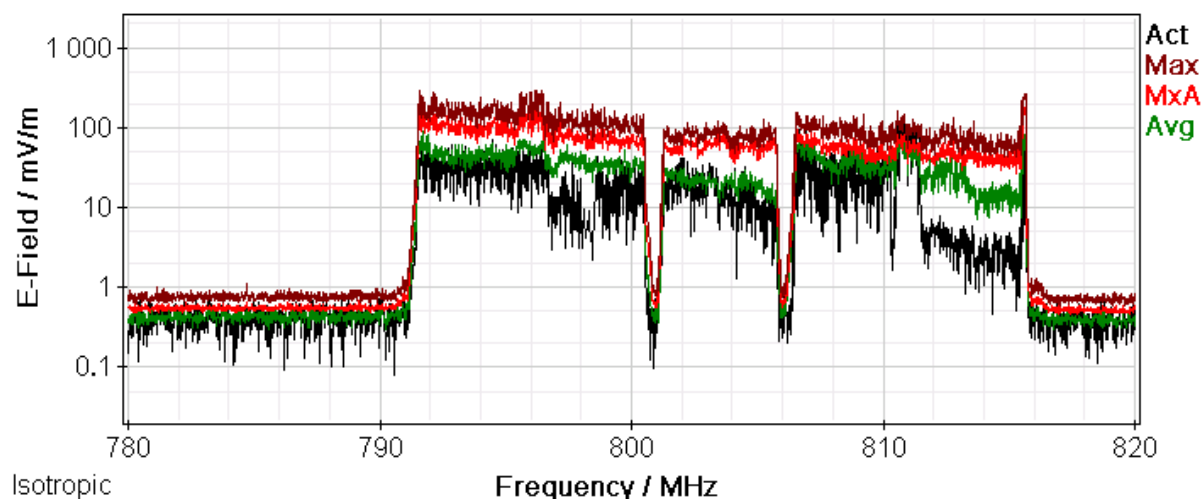
Rys. 8 Wyniki pomiarów selektywnych – zakres częstotliwości: 791,0 MHz – 821,0 MHz
