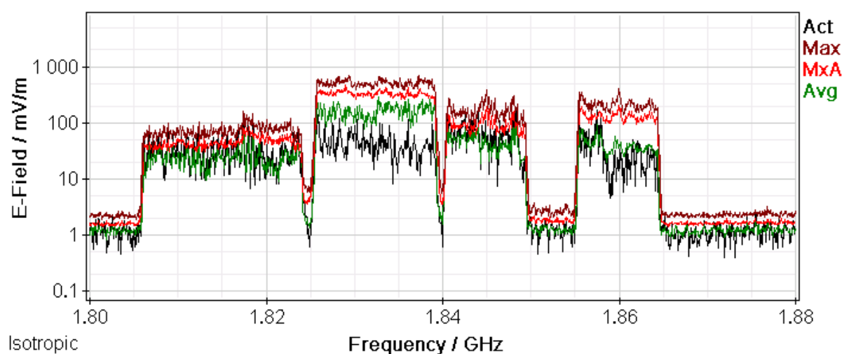
Rys. 10 Wyniki pomiarów selektywnych – zakres częstotliwości: 1805,1 MHz – 1879,9 MHz
