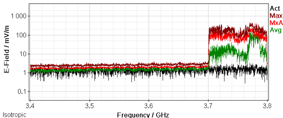
Rys. 13 Wyniki pomiarów selektywnych – zakres częstotliwości: 3400,0 MHz – 3800,0 MHz
