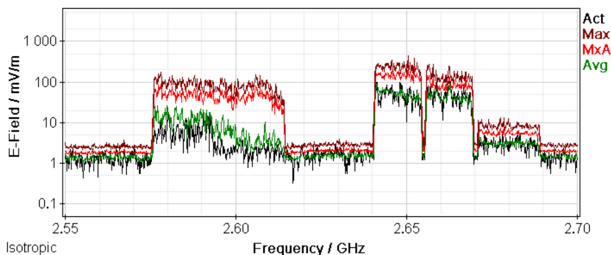
Rys. 12 Wyniki pomiarów selektywnych – zakres częstotliwości: 2570,0 MHz – 2690,0 MHz
