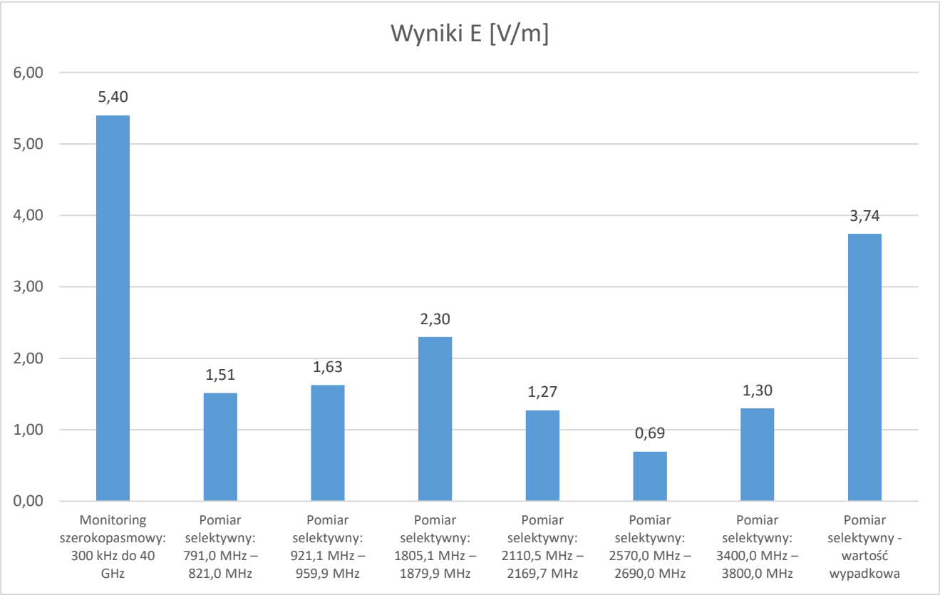
Rys. 14 Porównanie wyników monitoringu szerokopasmowego i pomiarów selektywnych
