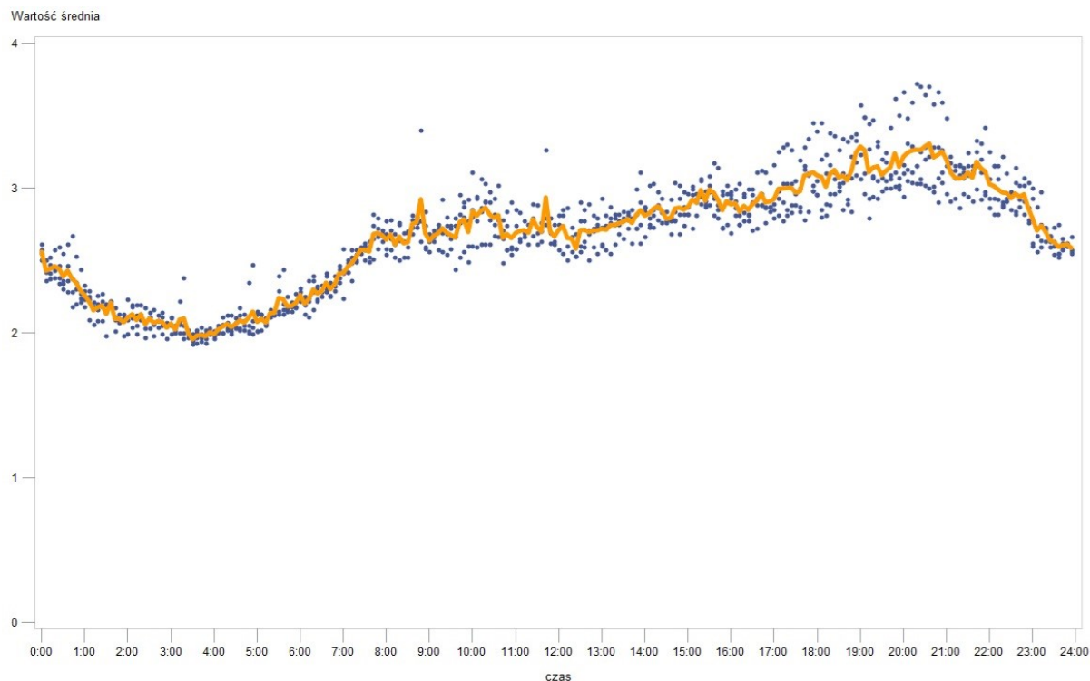
Rys. 6 Wyniki pomiarów – SP nr 16 w Siemianowicach – średnia za okres 24 godzin
