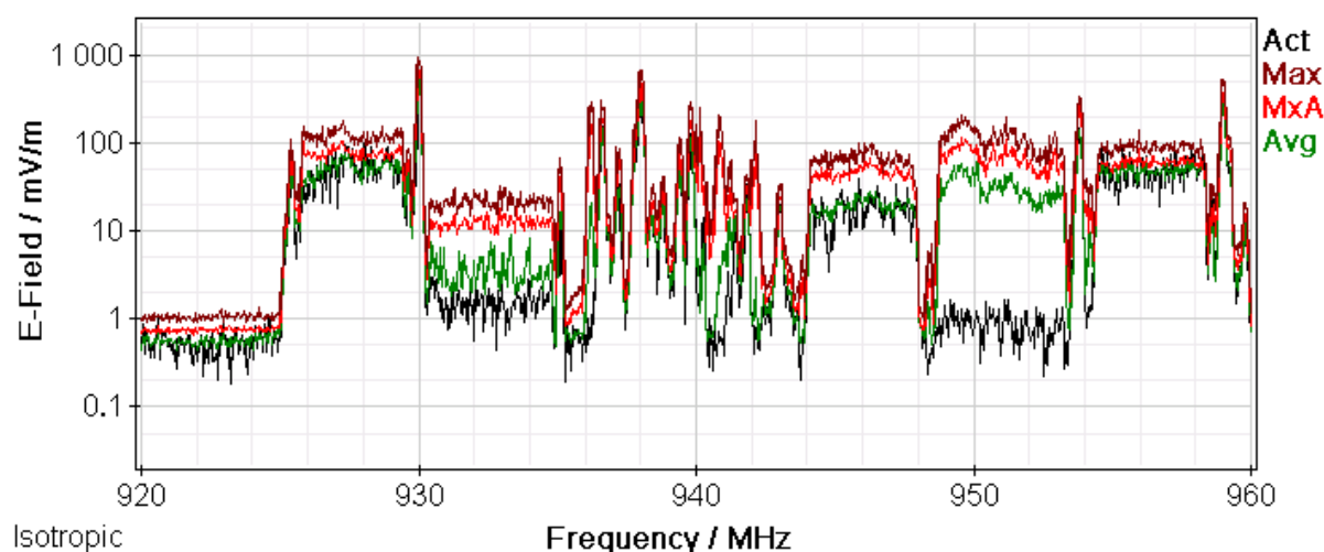
Rys. 9 Wyniki pomiarów selektywnych – zakres częstotliwości: 921,1 MHz – 959,9 MHz
