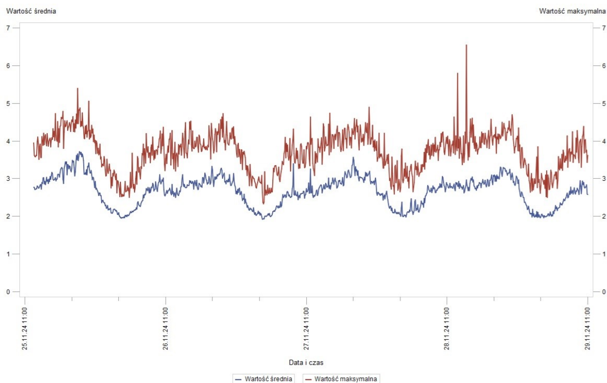
Rys. 5 Wyniki pomiarów – SP nr 16 w Siemianowicach w dniach 25.11.2024 r. – 29.11.2024 r. – wartość średnia i wartość maksymalna
