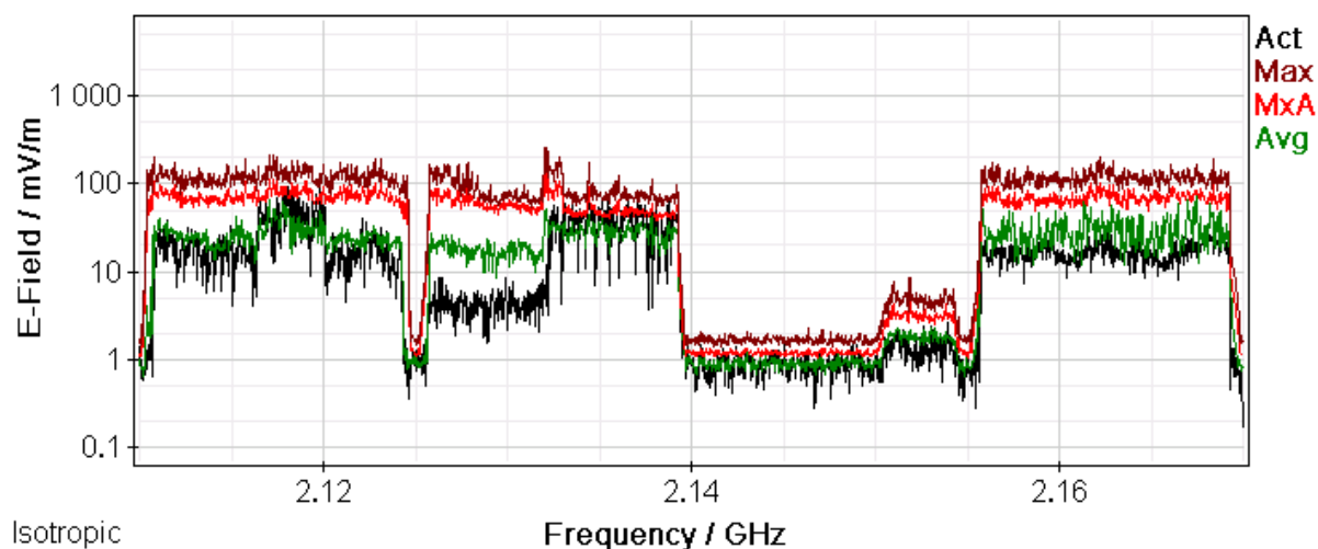
Rys. 11 Wyniki pomiarów selektywnych – zakres częstotliwości: 2110,5 MHz – 2169,7 MHz
