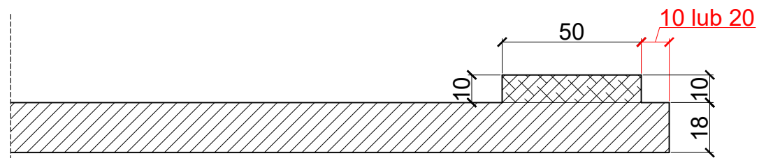
front - przekrój poprzeczny, wymiary w mm
