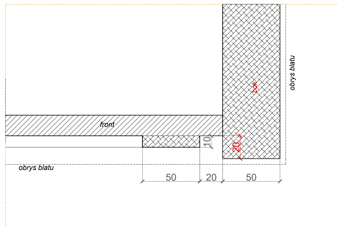
detal połączenia boków z frontami (rzut z góry), wymiary w mm.
