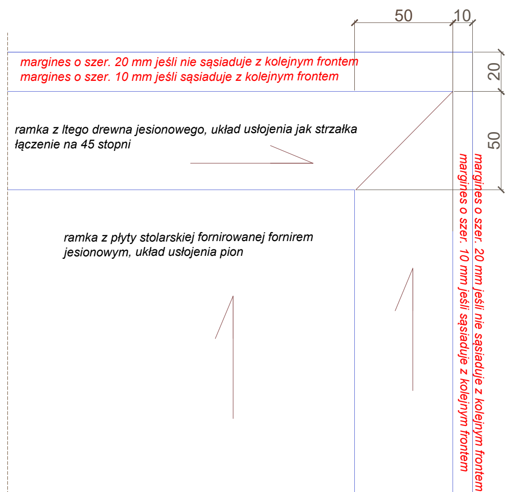
front - widok, wymiary w mm
