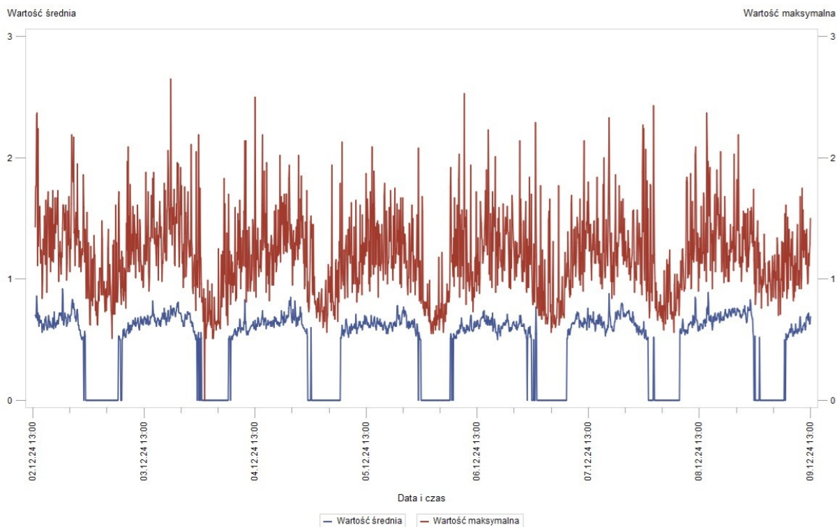
Rys. 6 Wyniki pomiarów – Zespół Szkół im. Staszica w Pile w dniach 2.12.2024 r. – 9.12.2024 r. – wartość średnia i wartość maksymalna
