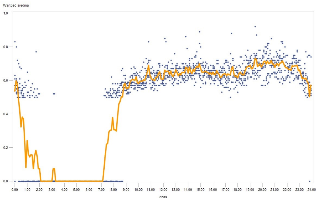
Rys. 7 Wyniki pomiarów – Zespół Szkół im. Staszica w Pile – średnia za okres 24 godzin
