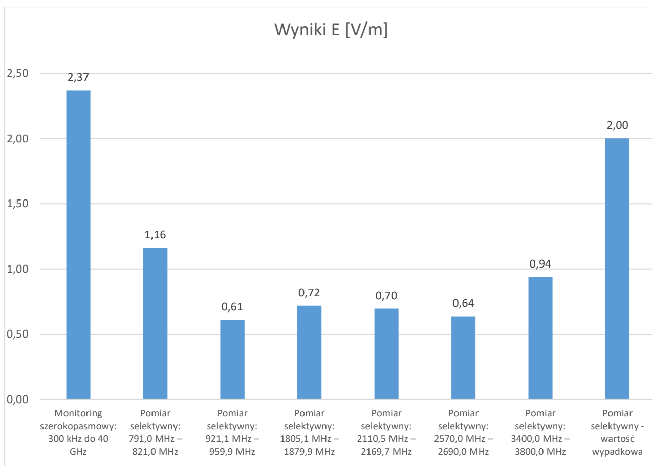
Rys. 15 Porównanie wyników monitoringu szerokopasmowego i pomiarów selektywnych
