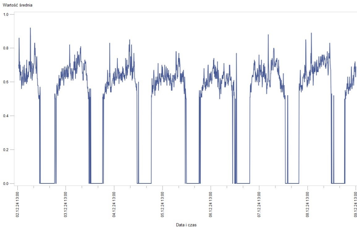
Rys. 5 Wyniki pomiarów – Zespół Szkół im. Staszica w Pile w dniach 2.12.2024 r. – 9.12.2024 r. – wartość średnia
