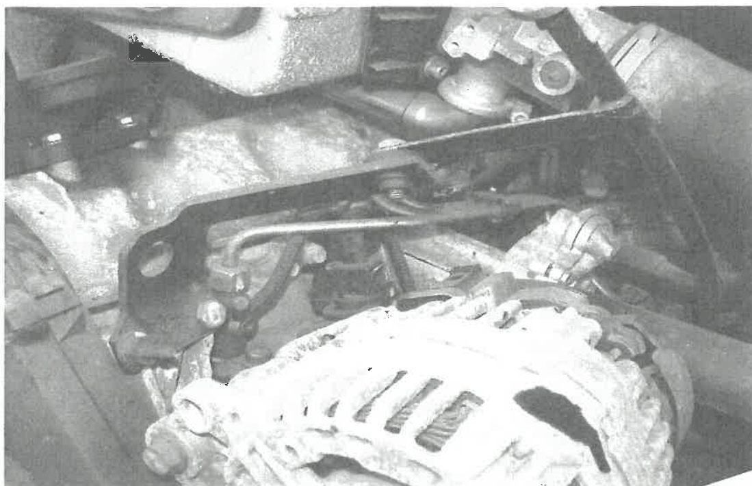
widok : osprzęt silnika wysokoprężnego
