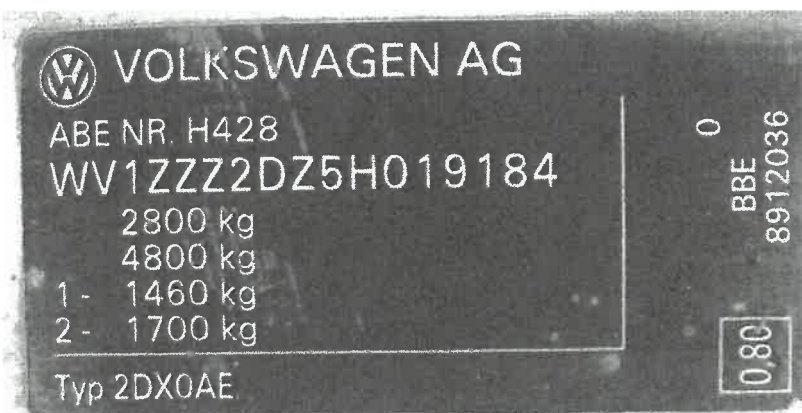
widok : tabliczka firmowa znamionowa identyfikacyjna
