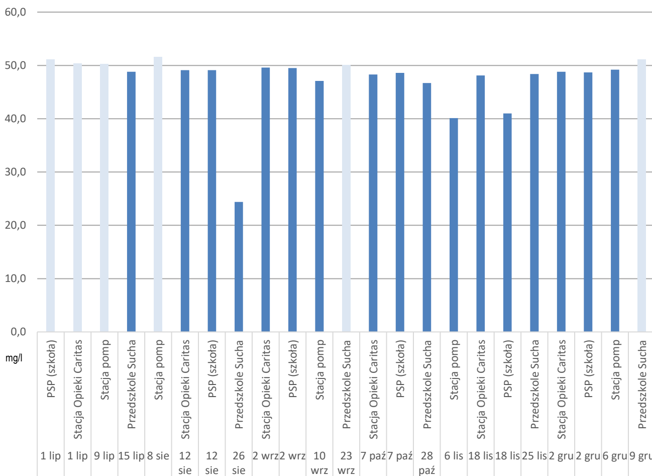
Wykres przedstawiający wartość stężenia azotanów w próbkach wody przeznaczonej do spożycia w II półroczu 2024 r.
