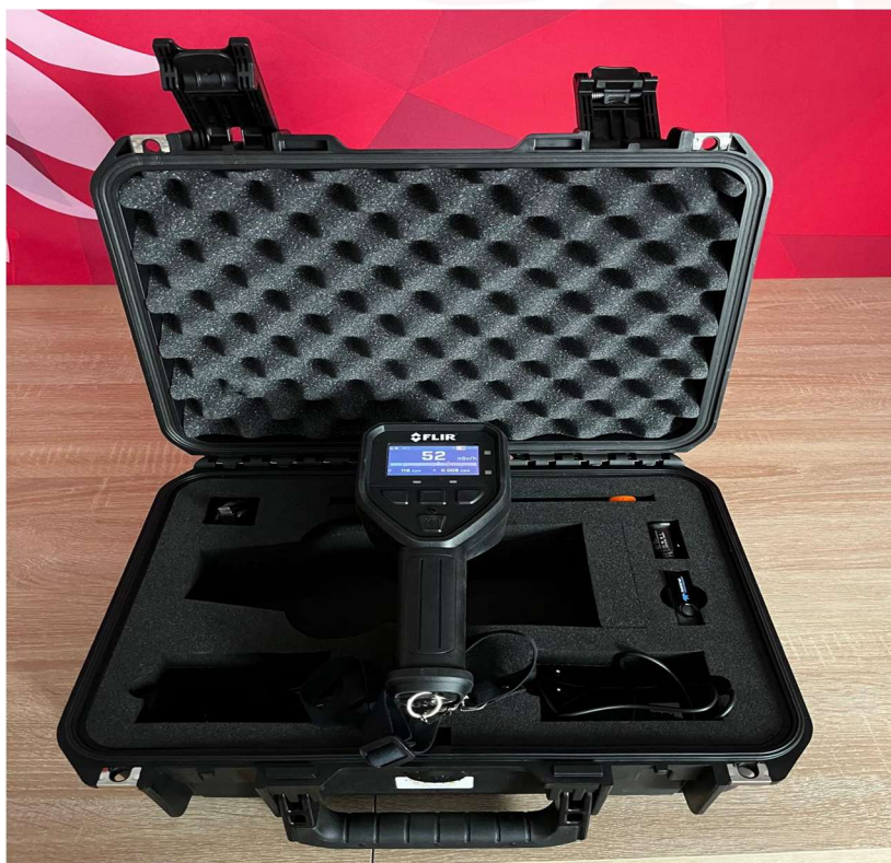
Fot. 26 Spektrometr promieniowania gamma
