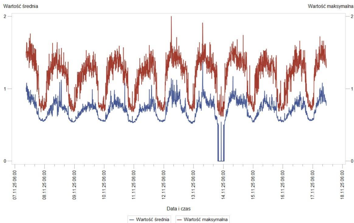
Rys. 6 Wyniki pomiarów – Szczecińskie Przedsiębiorstwo Autobusowe w dniach 7.11.2025 r. – 17.11.2025 r. – wartość średnia i wartość maksymalna
