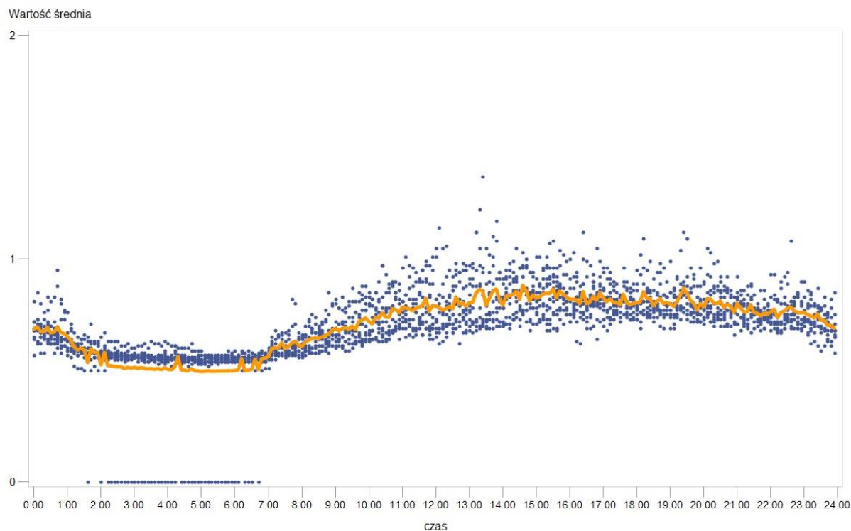
Rys. 7 Wyniki pomiarów – Szczecińskie Przedsiębiorstwo Autobusowe – średnia za okres 24 godzin
