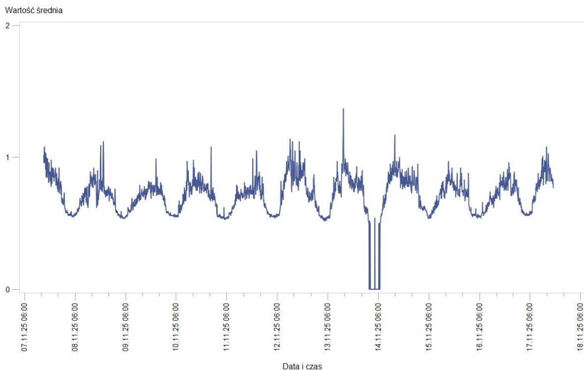
Rys. 5 Wyniki pomiarów – Szczecińskie Przedsiębiorstwo Autobusowe w dniach 7.11.2025 r. – 17.11.2025 r. – wartość średnia
