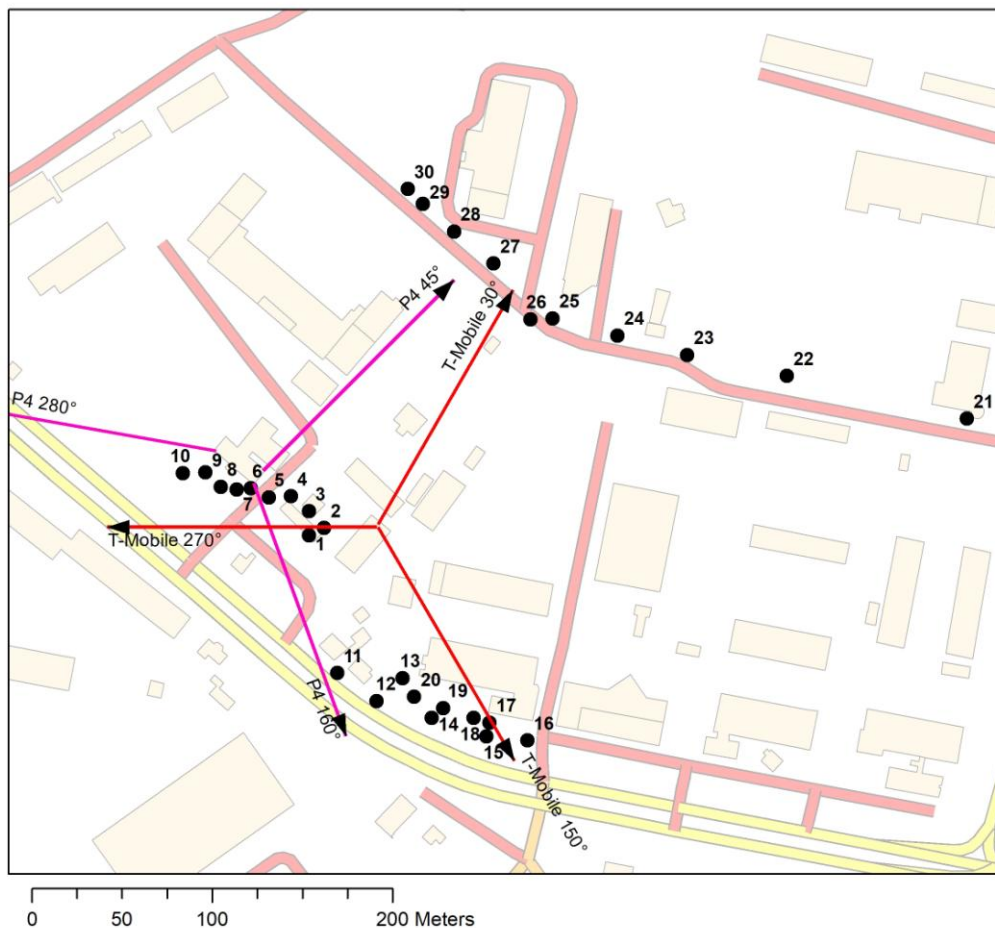
Rys. 1: Plan terenu, na którym znajdują się badana stacja bazowa
