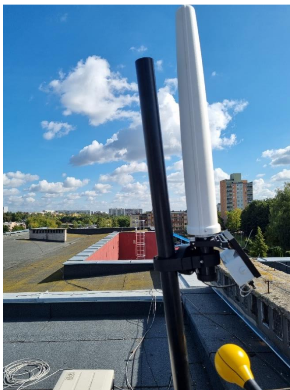
Rys. 8 Szkoła Podstawowa nr 51 w Lublinie – pomiary selektywne SRM-3600
