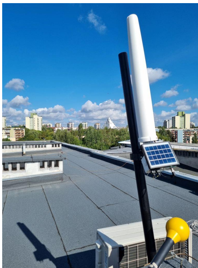
Rys. 2. Miejsce montażu SMS PEM – Szkoła Podstawowa nr 51 w Lublinie
