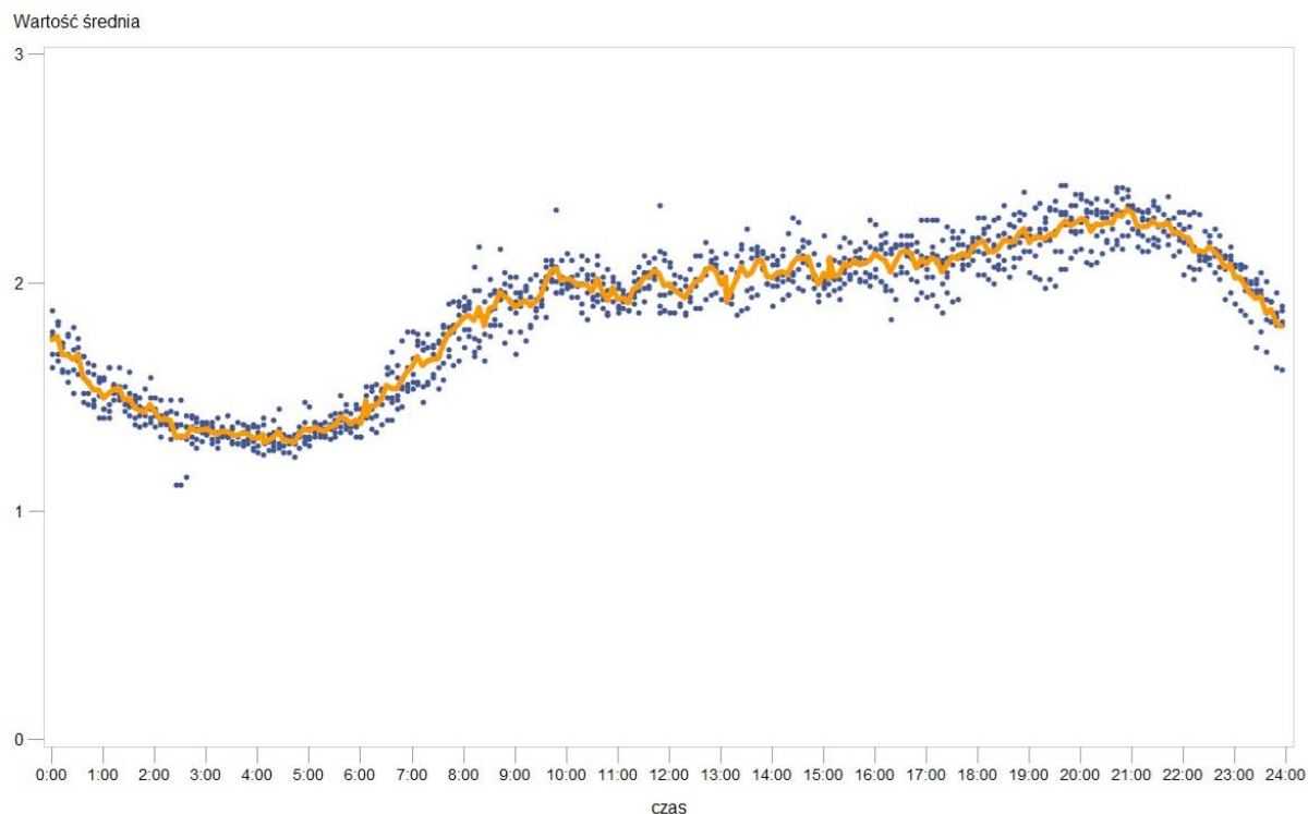
Rys. 7 Wyniki pomiarów – Szkoła Podstawowa nr 51 w Lublinie – średnia za okres 24 godzin
