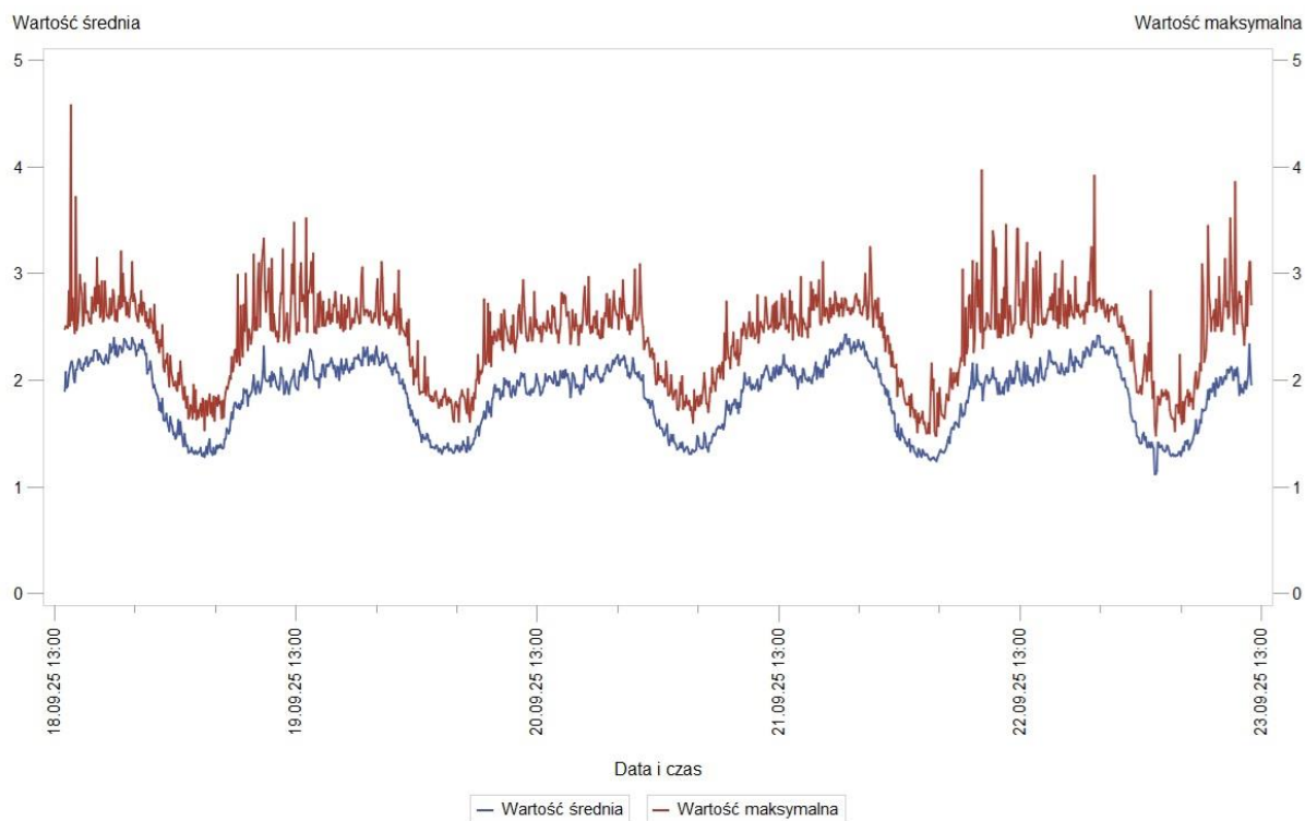
Rys. 6 Wyniki pomiarów – Szkoła Podstawowa nr 51 w Lublinie w dniach 18.09.2025 r. – 23.09.2025 r. – wartość średnia i wartość maksymalna
