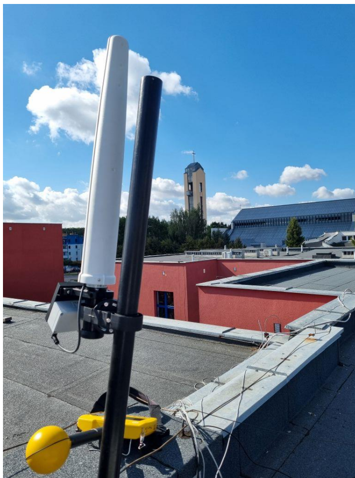
Rys. 3 Miejsce montażu SMS PEM – Szkoła Podstawowa nr 51 w Lublinie
