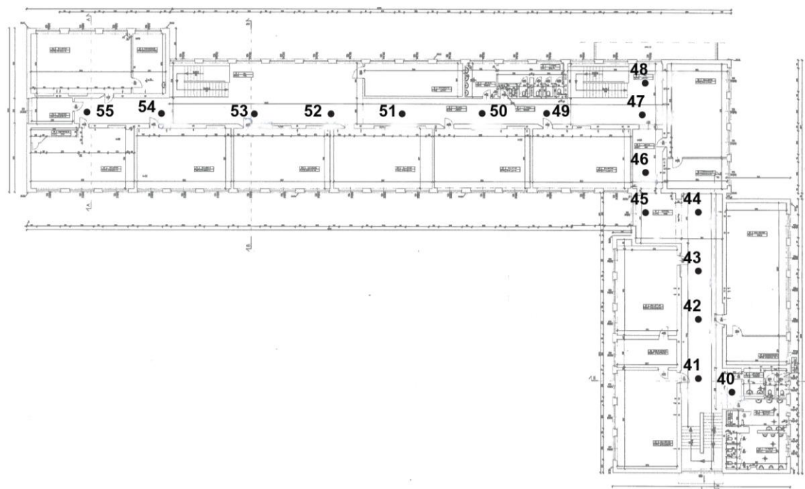
Rys. 1d: Plan rozmieszczenia punktów pomiarowych – II piętro
