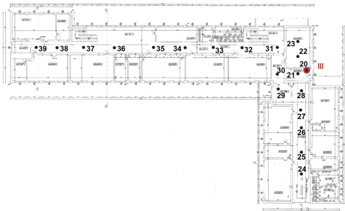
Rys. 1c: Plan rozmieszczenia punktów pomiarowych – I piętro kolorem czerwonym oznaczono lokalizację punktu dostępowego
