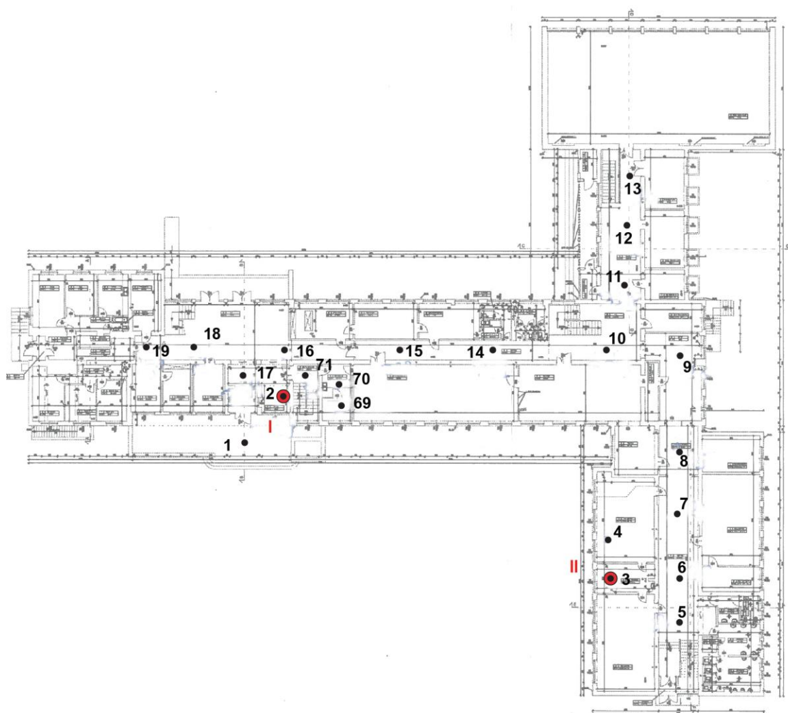
Rys. 1b: Plan rozmieszczenia punktów pomiarowych – parter kolorem czerwonym oznaczono lokalizację punktów dostępowych
