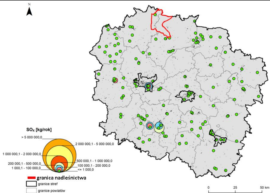
Ryc. 39 Lokalizacja punktowych źródeł emisji \text{SO}_x na obszarze województwa kujawsko-pomorskiego [źródło danych: KOBIZE/IOŚ-PIB].
