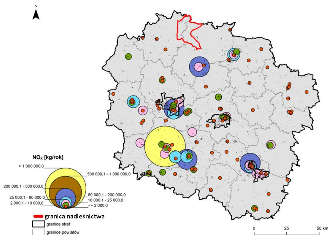
Ryc. 40 Lokalizacja punktowych źródeł emisji \text{NO}_x na obszarze województwa kujawsko-pomorskiego [źródło danych: KOBIZE/IOŚ-PIB].
