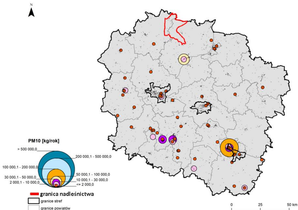
Ryc. 41 Lokalizacja punktowych źródeł emisji PM10 na obszarze województwa kujawsko-pomorskiego [źródło danych: KOBIZE/IOŚ-PIB].
