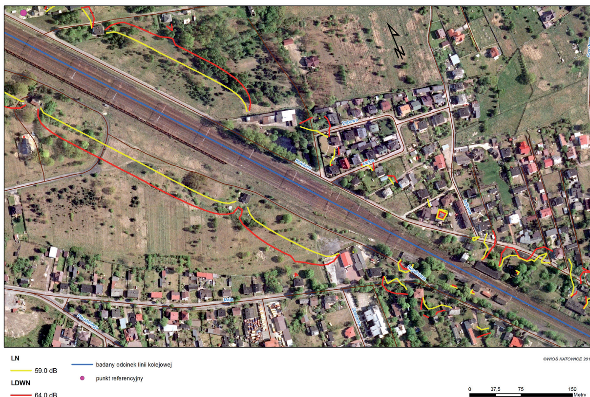
Mapa 3. Fragment mapy akustycznej dla wskaźnika oceny hałasu L_{DWN} oraz wskaźnika L_N w rejonie badań RB1 – ul. Kolejowa, Poraj 2013 rok
