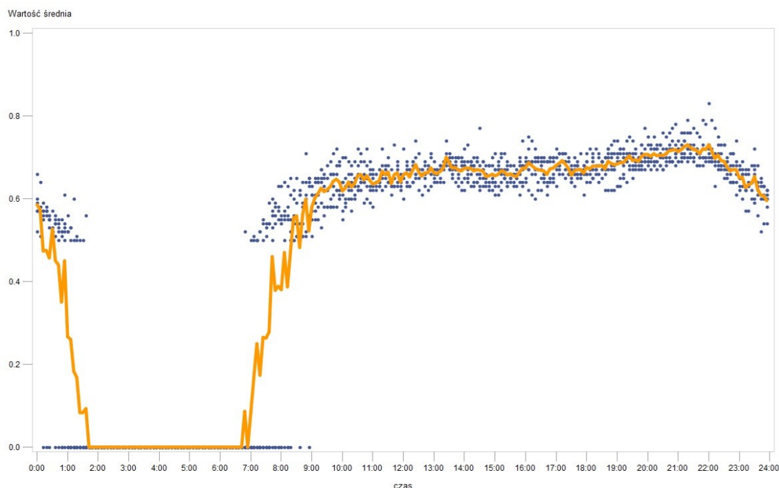
Rys. 7 Wyniki pomiarów – ZSET w Gdyni – średnia za okres 24 godzin
