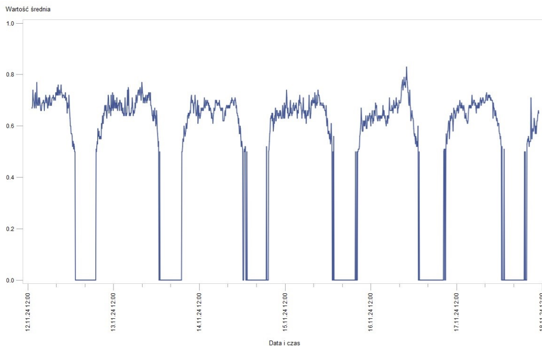
Rys. 5 Wyniki pomiarów – ZSET w Gdyni w dniach 12.11.2024 r. – 18.11.2024 r. – wartość średnia
