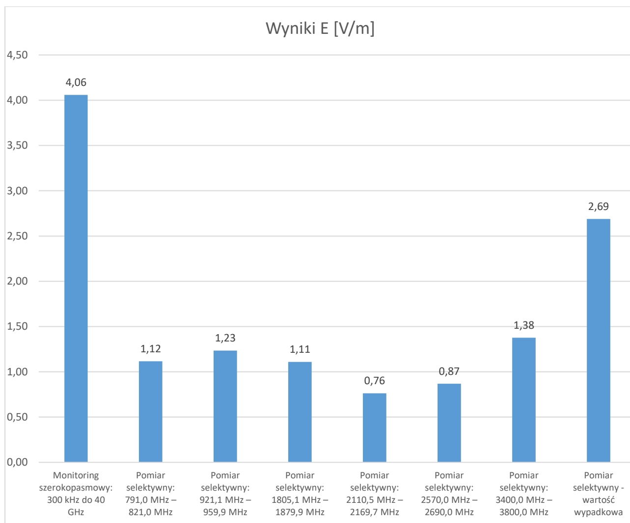
Rys. 15 Porównanie wyników monitoringu szerokopasmowego i pomiarów selektywnych
