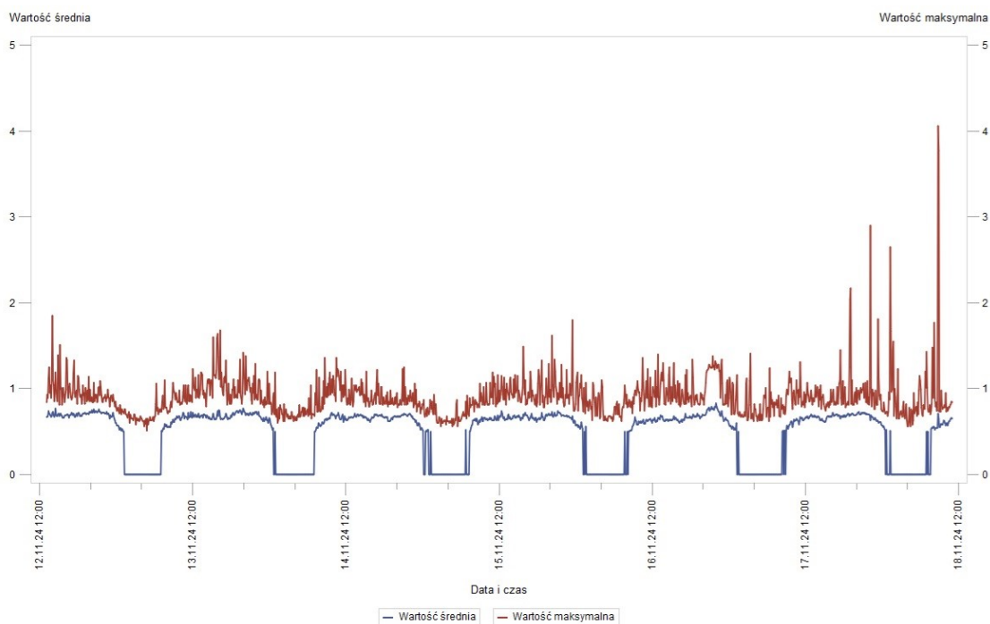
Rys. 6 Wyniki pomiarów – ZSET w Gdyni w dniach 12.11.2024 r. – 18.11.2024 r. – wartość średnia i wartość maksymalna
