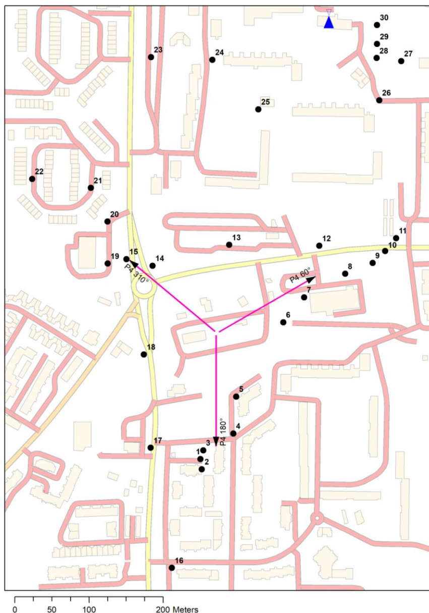
Rys. 1: Plan terenu, na którym znajdują się badane stacje bazowe
