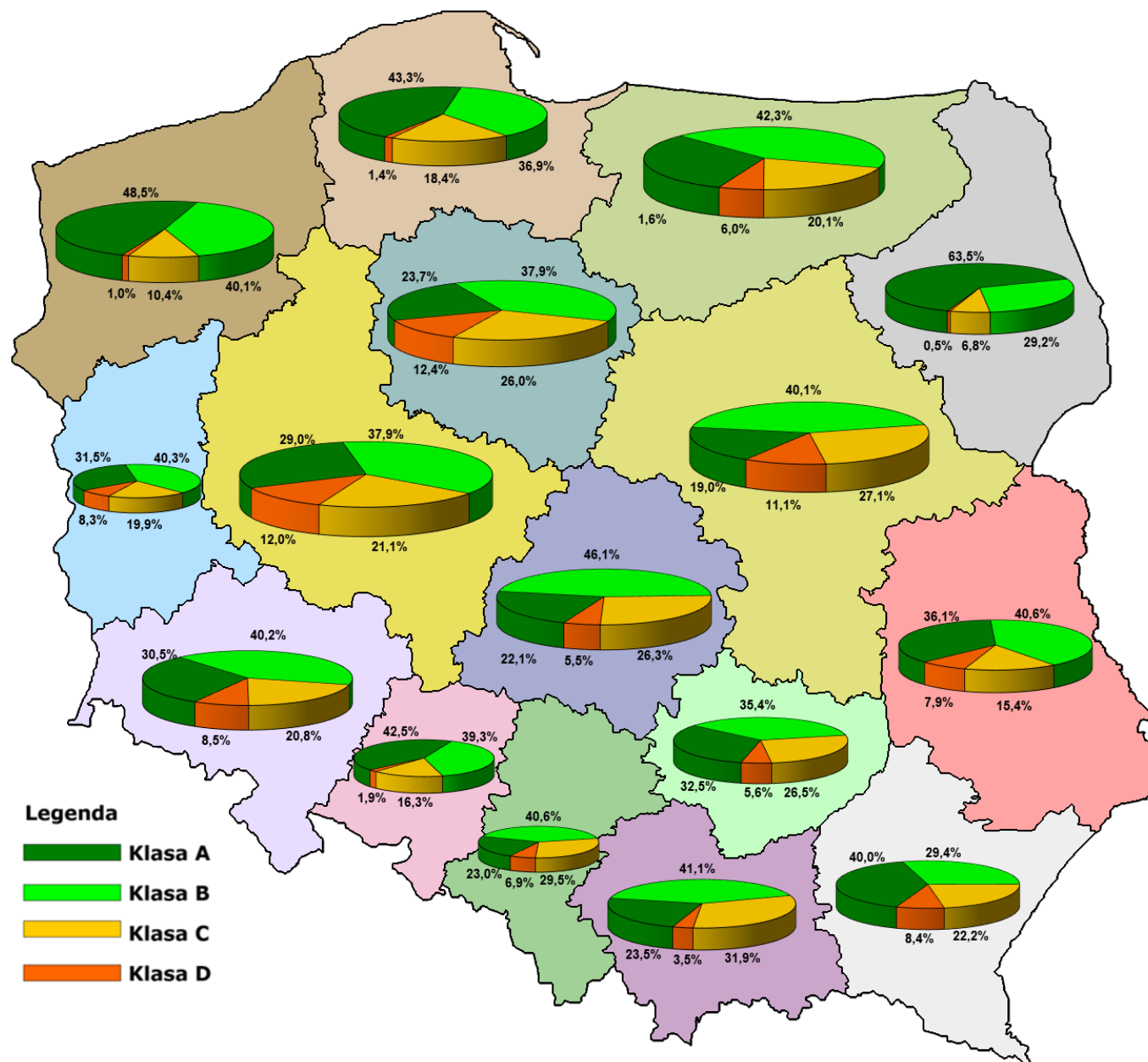
Rysunek 7. Stan techniczny pod względem parametru: współczynnik tarcia
