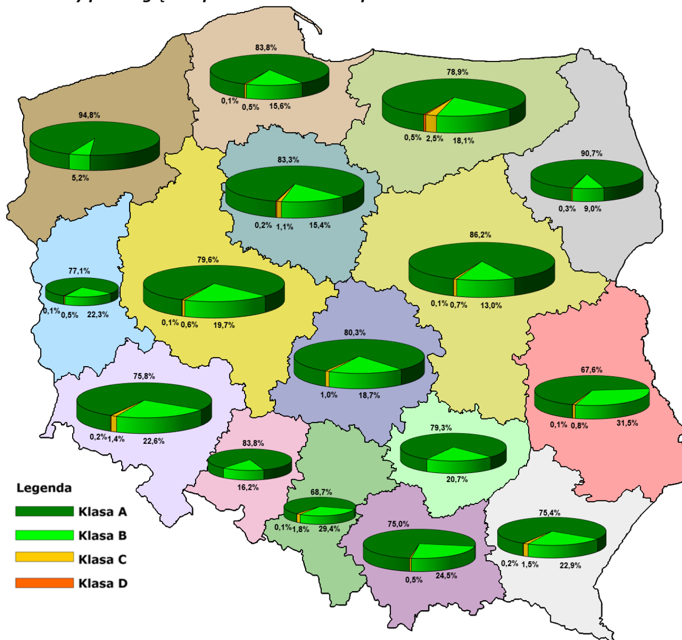
Rysunek 6. Stan techniczny pod względem parametru: równość podłużna
