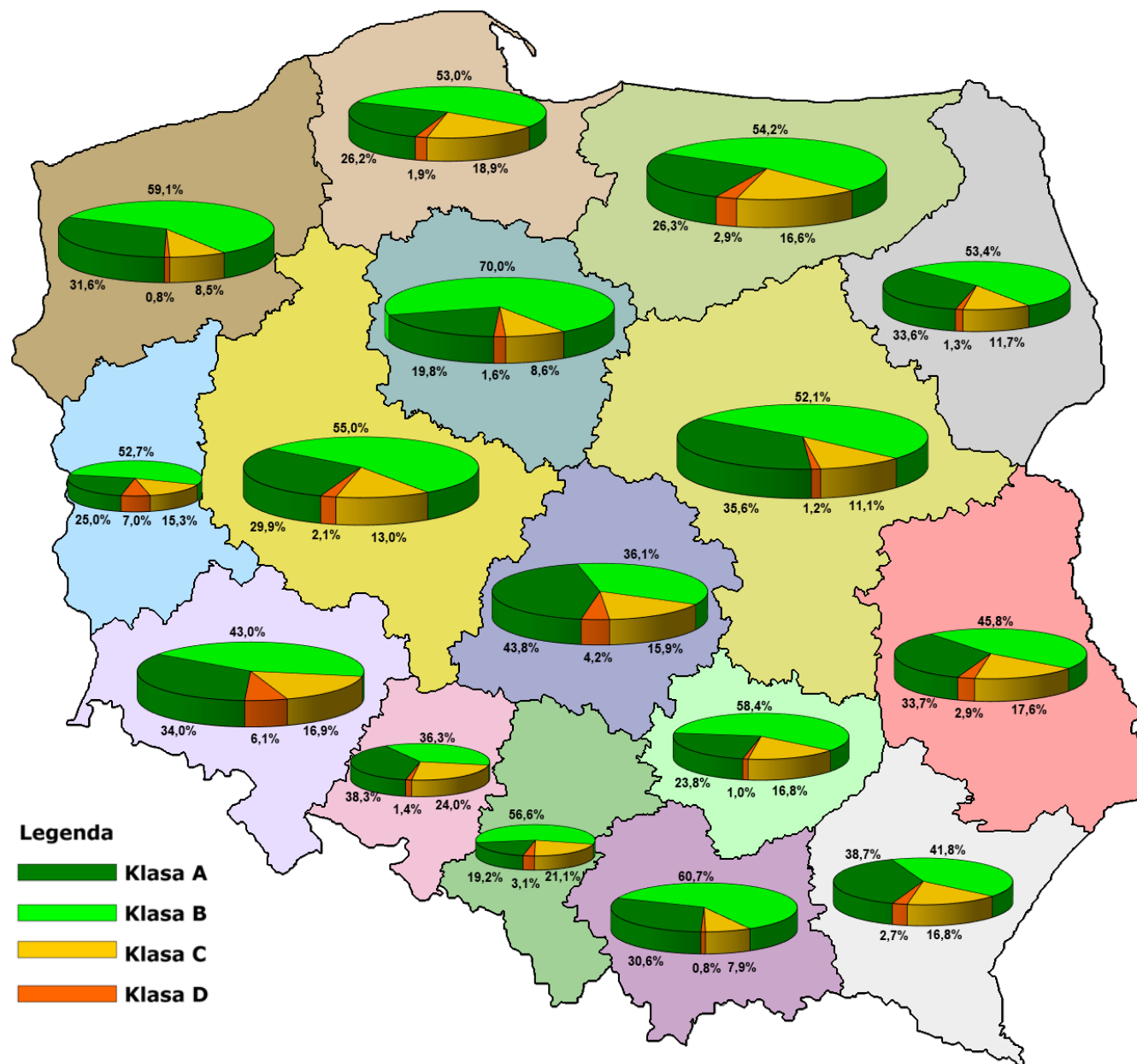
Rysunek 1. Stan techniczny pod względem parametru: stan spękań
