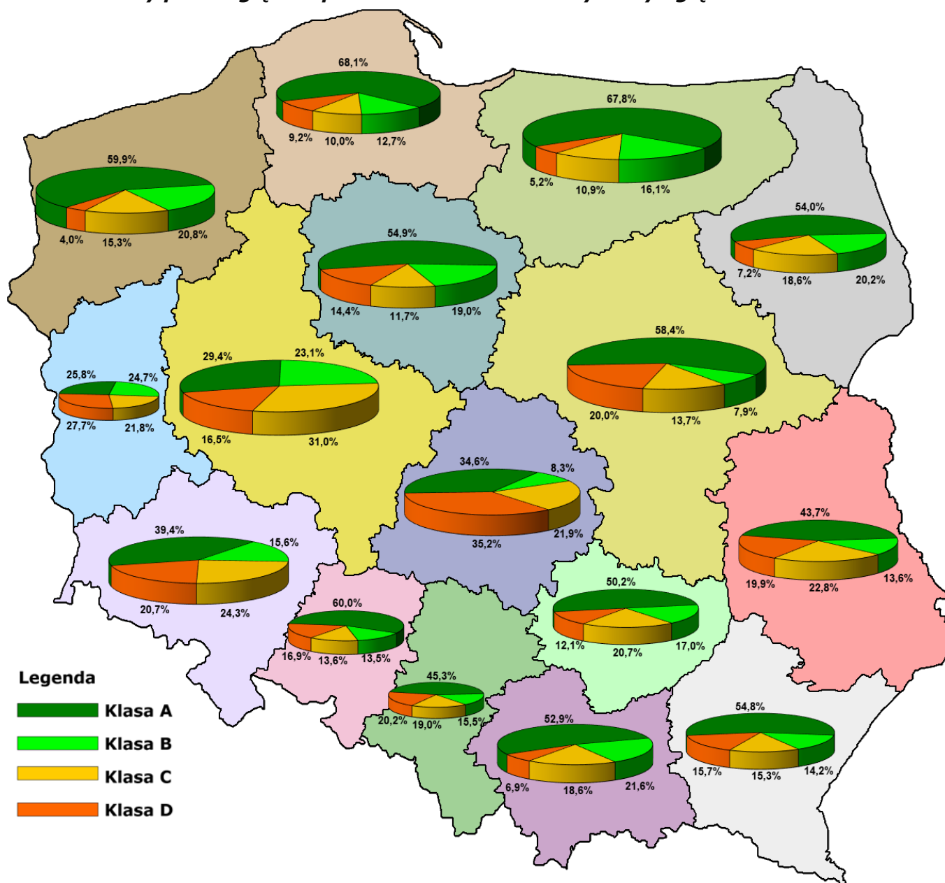
Rysunek 3. Stan techniczny pod względem parametru: wskaźnik krzywizny ugięcia
