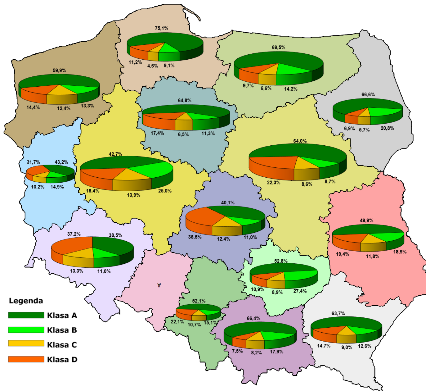
Rysunek 2. Stan techniczny pod względem parametru: wskaźnik ugięć nawierzchni
