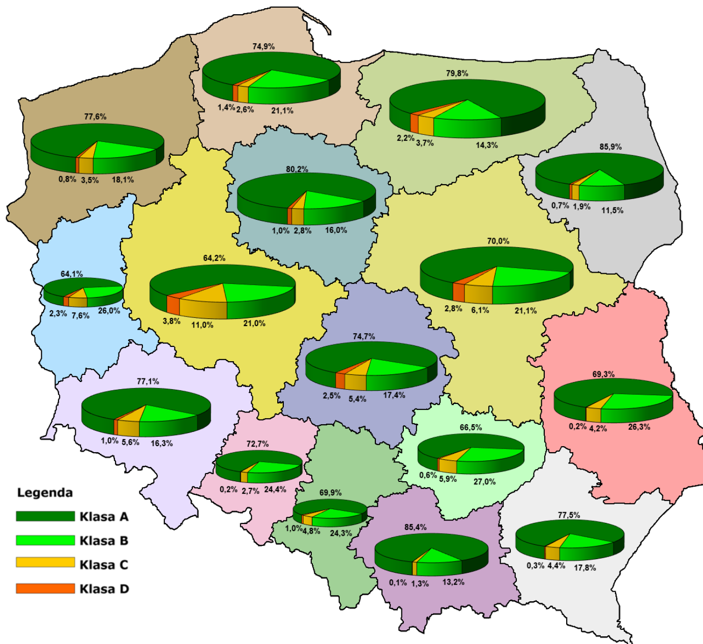
Rysunek 5. Stan techniczny pod względem parametru: koleiny
