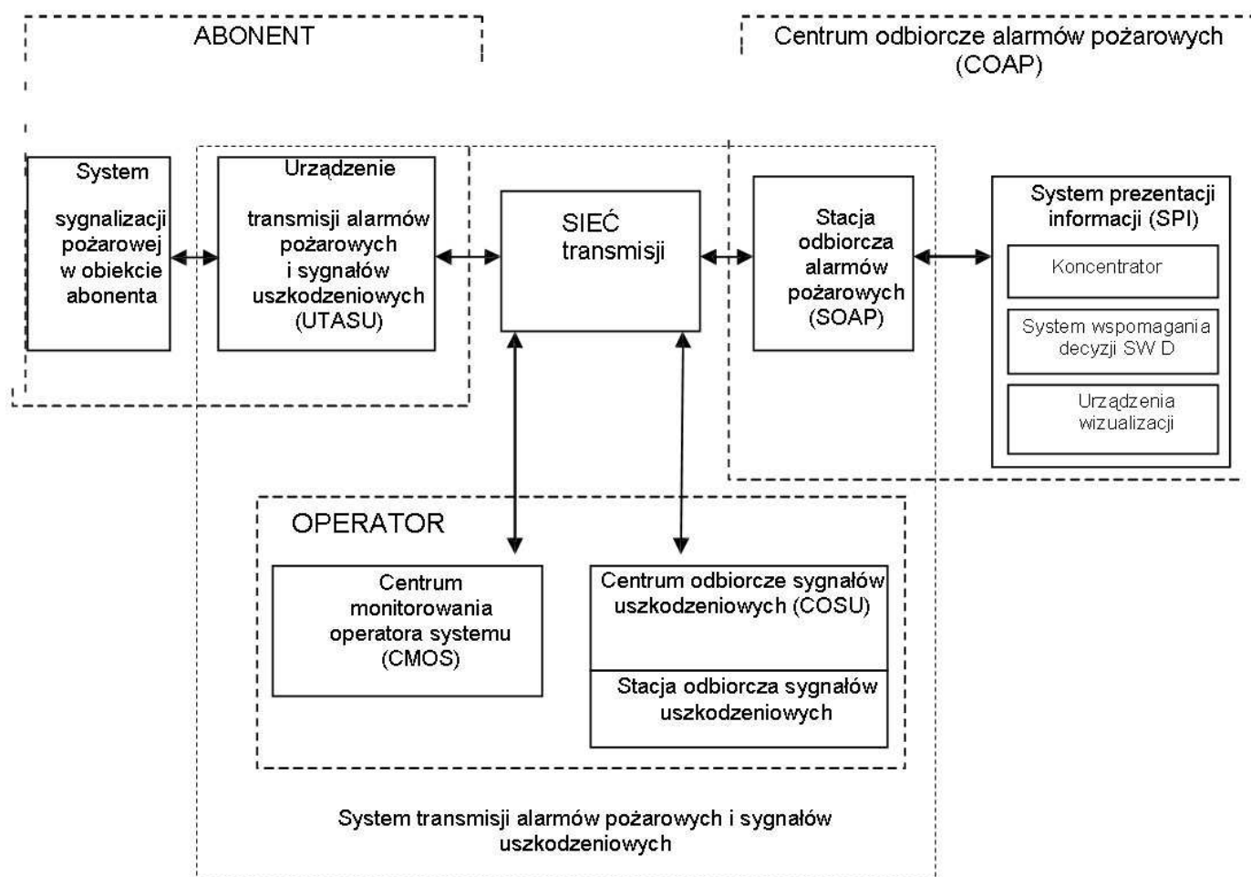
Rysunek 3. System transmisji alarmów pożarowych ze stacją pośredniczącą
