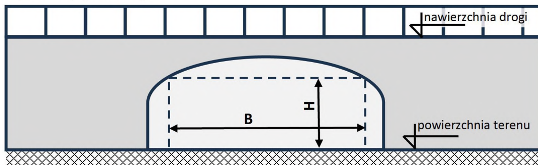
Rysunek 1: Wymiary przejścia dolnego dla zwierząt (B – szerokość, H – wysokość) – widok w przekroju poprzecznym przejścia
