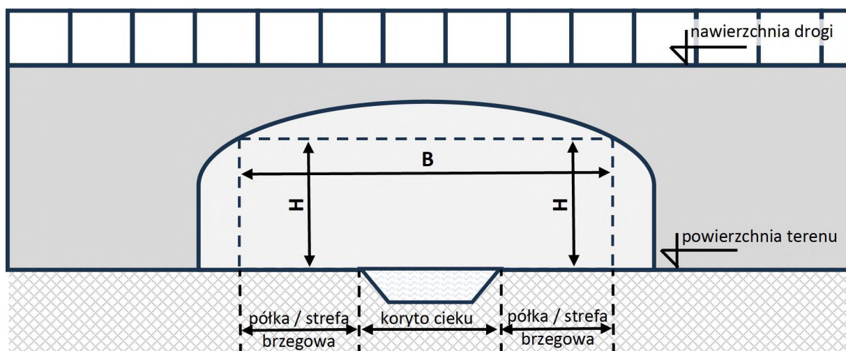
Rysunek 2: Wymiary przejścia dolnego dla zwierząt zintegrowanego z ciekim (B – szerokość, H – wysokość) – widok w przekroju poprzecznym przejścia
