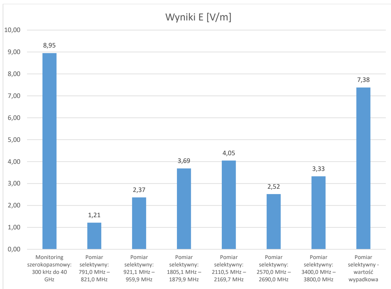
Rys. 16 Porównanie wyników monitoringu szerokopasmowego i pomiarów selektywnych
