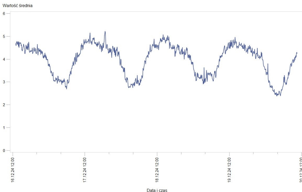
Rys. 6 Wyniki pomiarów – Rynek 1 w dniach 16.12.2024 r. – 20.12.2024 r. – wartość średnia
