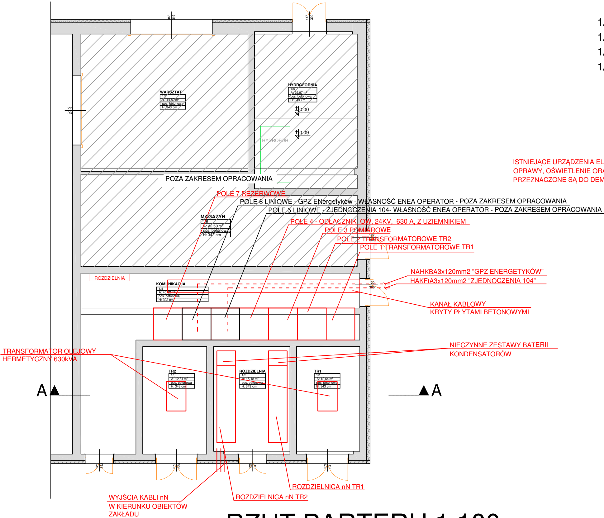
RZUT PARTERU 1:100
