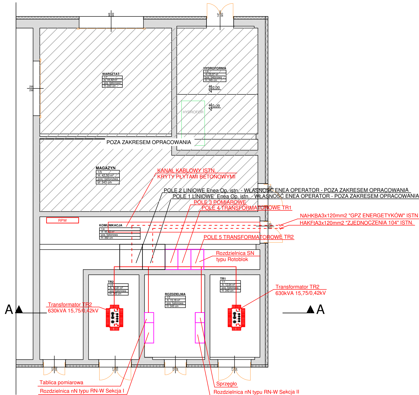
RZUT PARTERU 1:100
