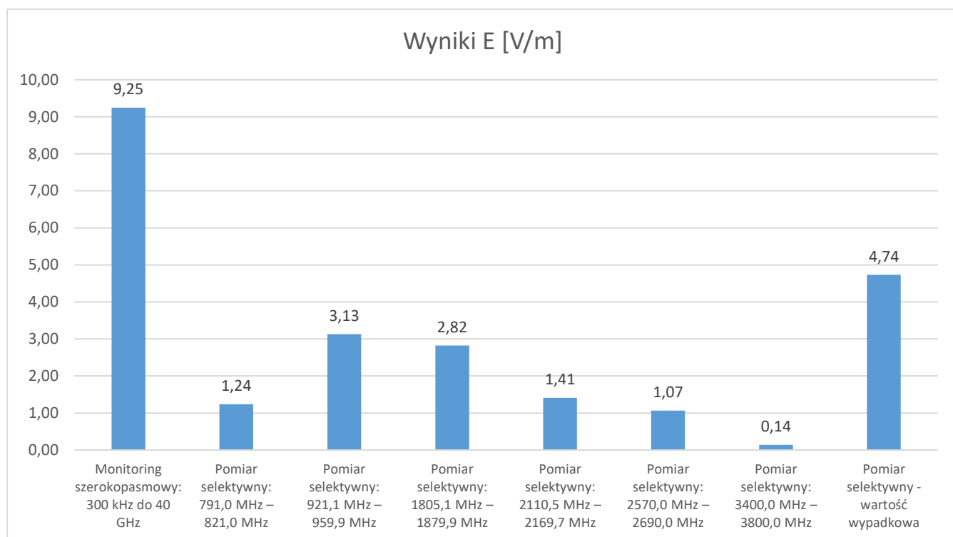
Rys. 15 Porównanie wyników monitoringu szerokopasmowego i pomiarów selektywnych
