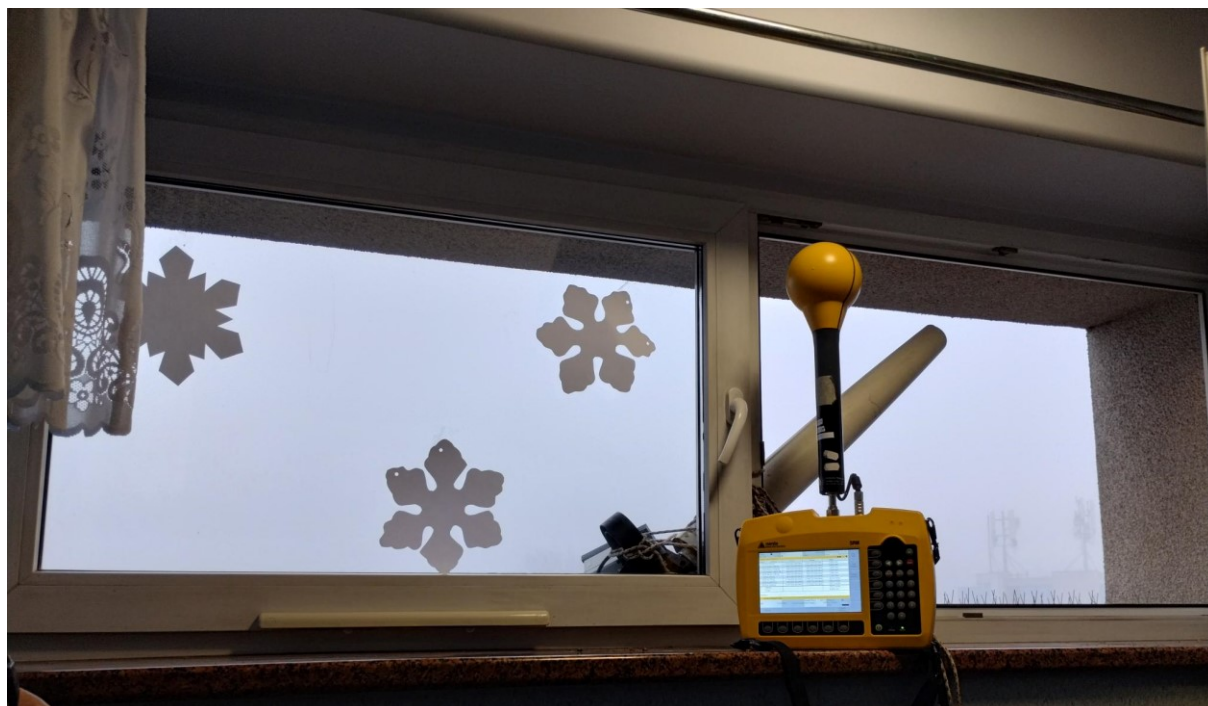
Rys. 2 Miejsce montażu SMS PEM – Hala Wałbrzyskich Mistrzów – widok na SBTK
