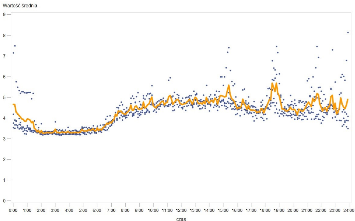
Rys. 7 Wyniki pomiarów – Hala Wałbrzyskich Mistrzów – średnia za okres 24 godzin
