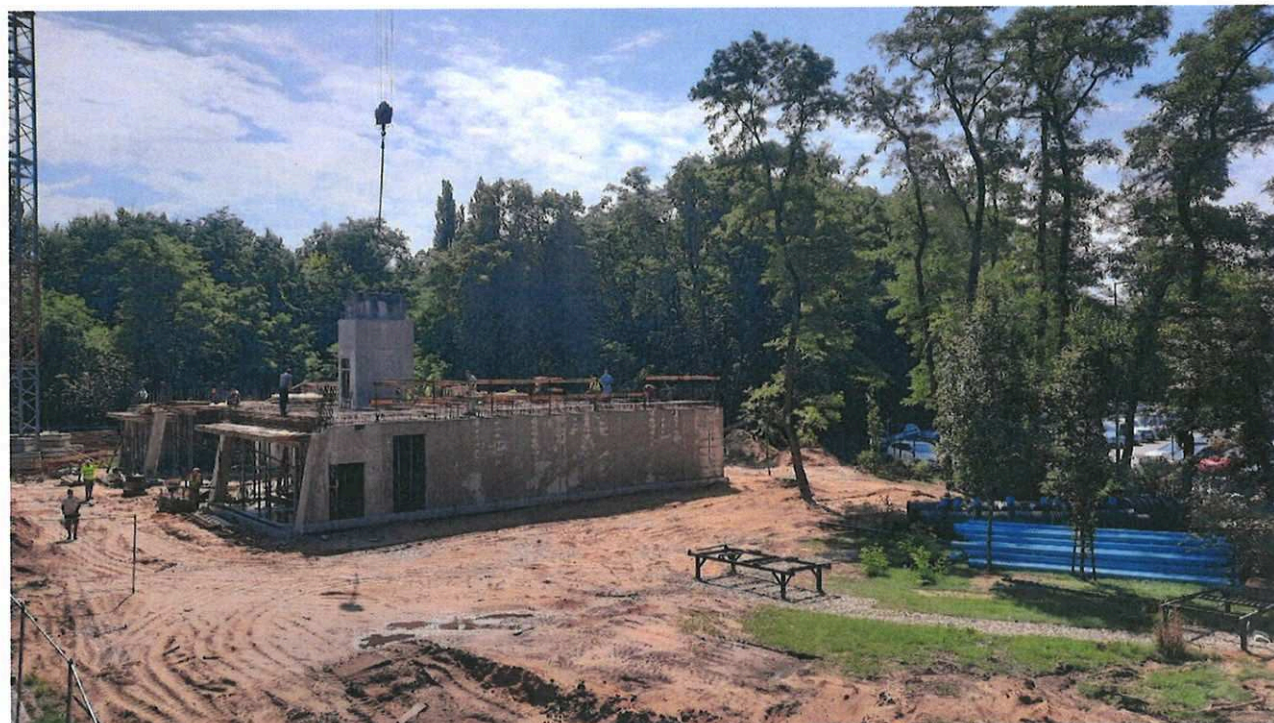
Fot. 11. Zamknięcie pierwszej kondygnacji Budynku B.
