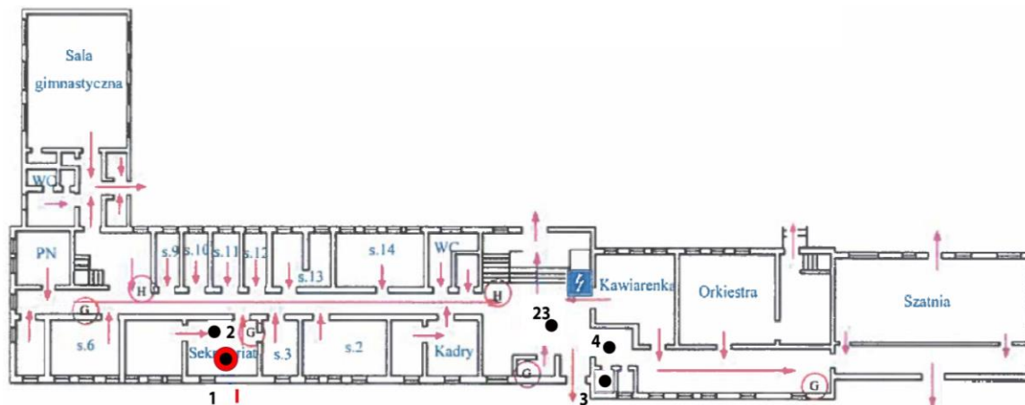
Rys. 1a: Plan rozmieszczenia punktów pomiarowych, kolorem czerwonym oznaczono lokalizację punktów dostępowych.
