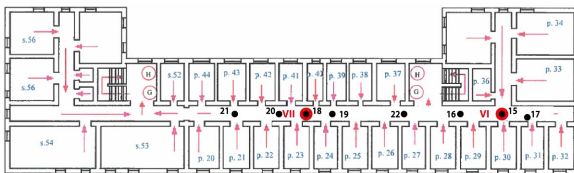
Rys. 1d: Plan rozmieszczenia punktów pomiarowych, kolorem czerwonym oznaczono lokalizację punktów dostępowych
