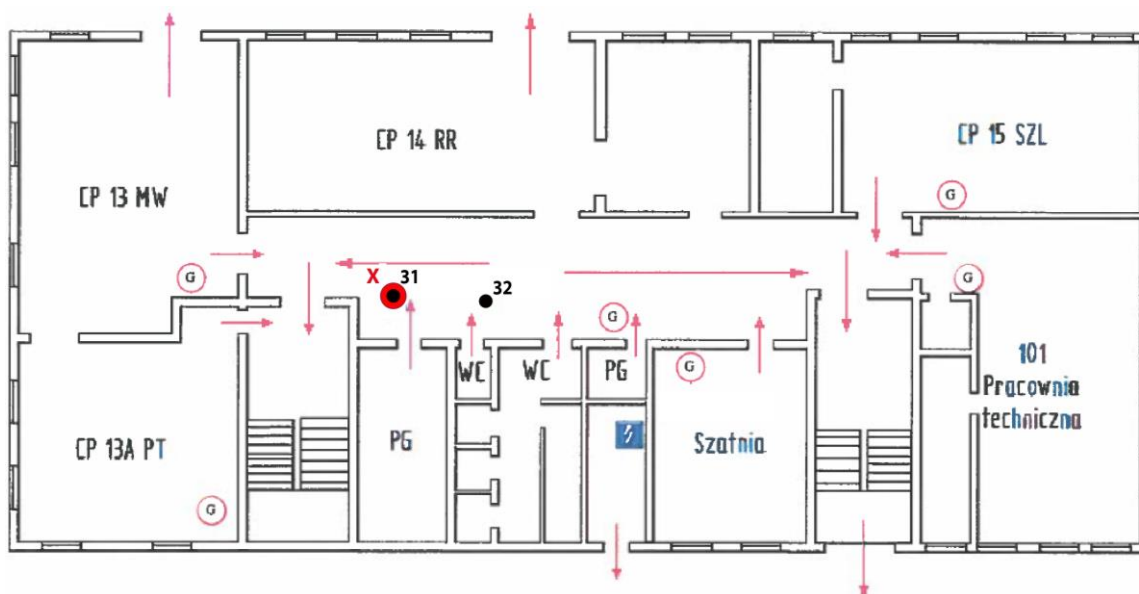
Rys. 1f: Plan rozmieszczenia punktów pomiarowych, kolorem czerwonym oznaczono lokalizację punktów dostępowych
