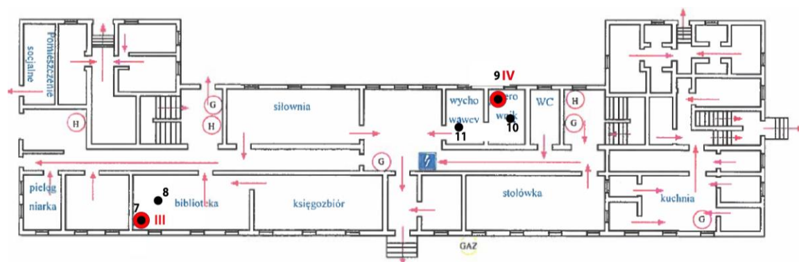
Rys. 1c: Plan rozmieszczenia punktów pomiarowych, kolorem czerwonym oznaczono lokalizację punktów dostępowych
