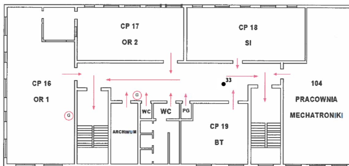
Rys. 1g: Plan rozmieszczenia punktów pomiarowych, kolorem czerwonym oznaczono lokalizację punktów dostępowych
