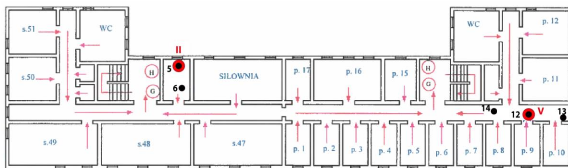
Rys. 1b: Plan rozmieszczenia punktów pomiarowych, kolorem czerwonym oznaczono lokalizację punktów dostępowych
