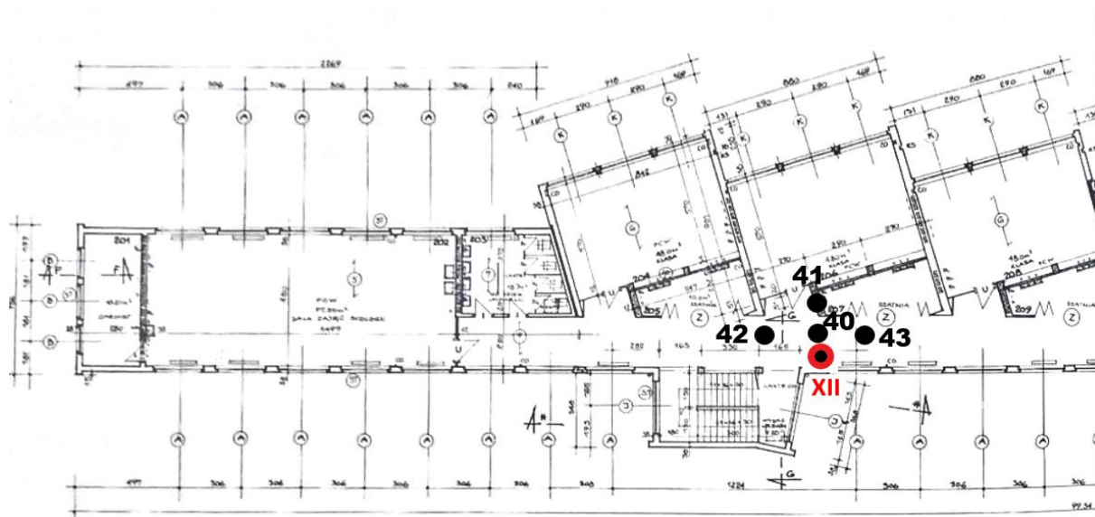
Rys. 1e: Plan rozmieszczenia punktów pomiarowych – 2 piętro (część 1), kolorem czerwonym oznaczono lokalizację punktów dostępowych
