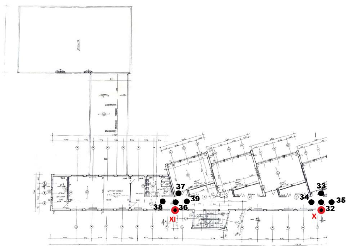
Rys. 1d: Plan rozmieszczenia punktów pomiarowych – I piętro (część 2), kolorem czerwonym oznaczono lokalizację punktów dostępowych
