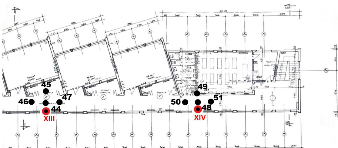
Rys. 1e: Plan rozmieszczenia punktów pomiarowych – 2 piętro (część 1), kolorem czerwonym oznaczono lokalizację punktów dostępowych
