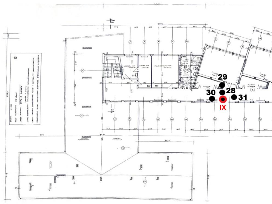
Rys. 1c: Plan rozmieszczenia punktów pomiarowych – I piętro (część 1), kolorem czerwonym oznaczono lokalizację punktów dostępowych
