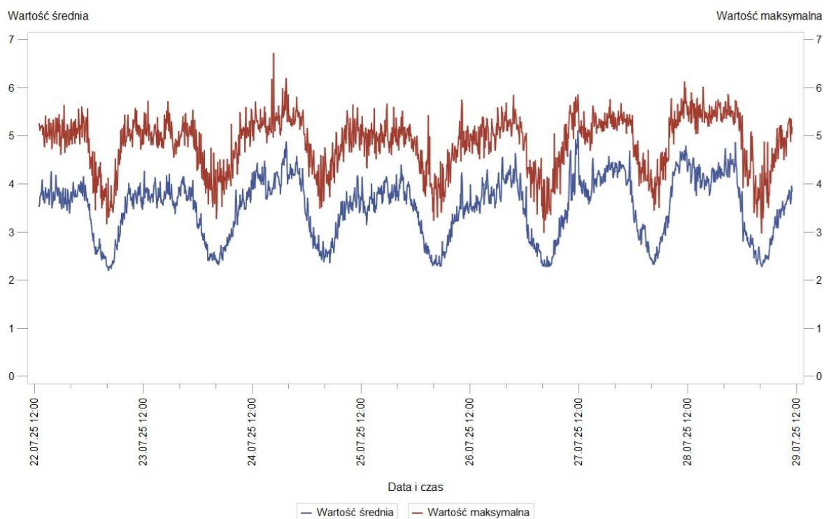
Rys. 6 Wyniki pomiarów – Szkoła Podstawowa nr 1 w Tarnowie w dniach 22.07.2025 r. – 29.07.2025 r. – wartość średnia i wartość maksymalna
