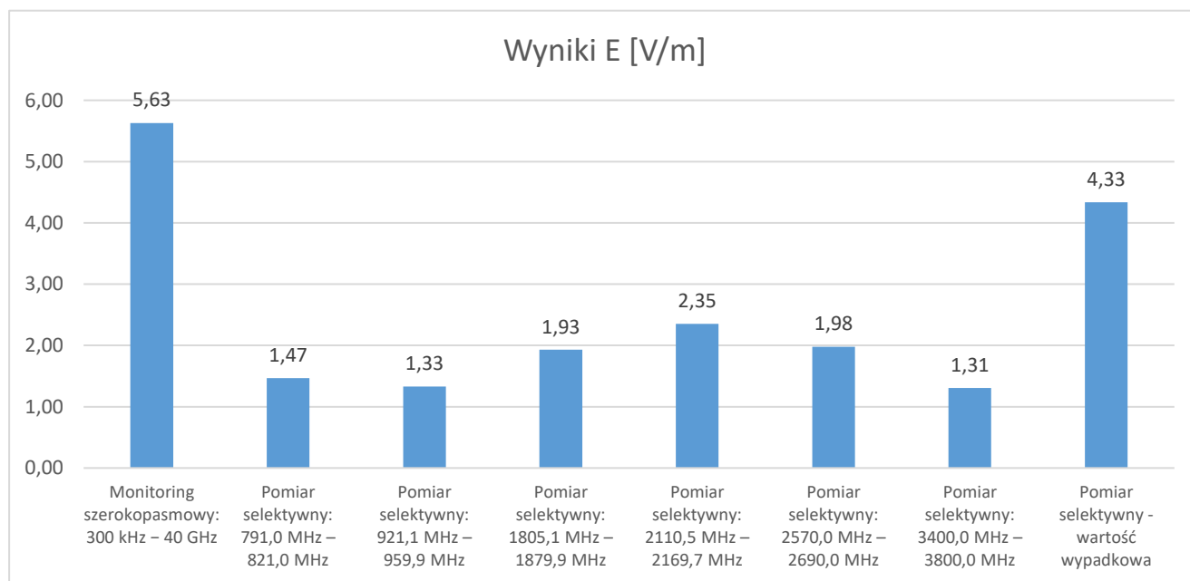
Rys. 15 Porównanie wyników monitoringu szerokopasmowego i pomiarów selektywnych
