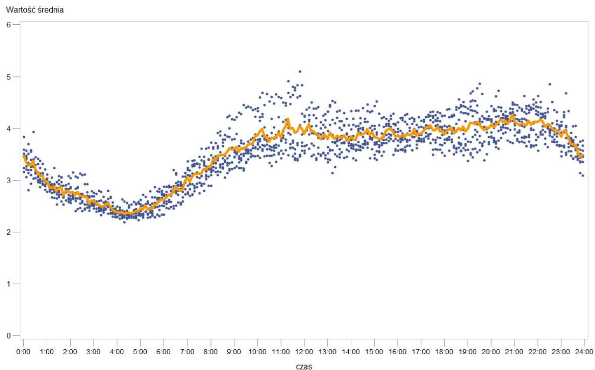
Rys. 7 Wyniki pomiarów – Szkoła Podstawowa nr 1 w Tarnowie – średnia za okres 24 godzin
