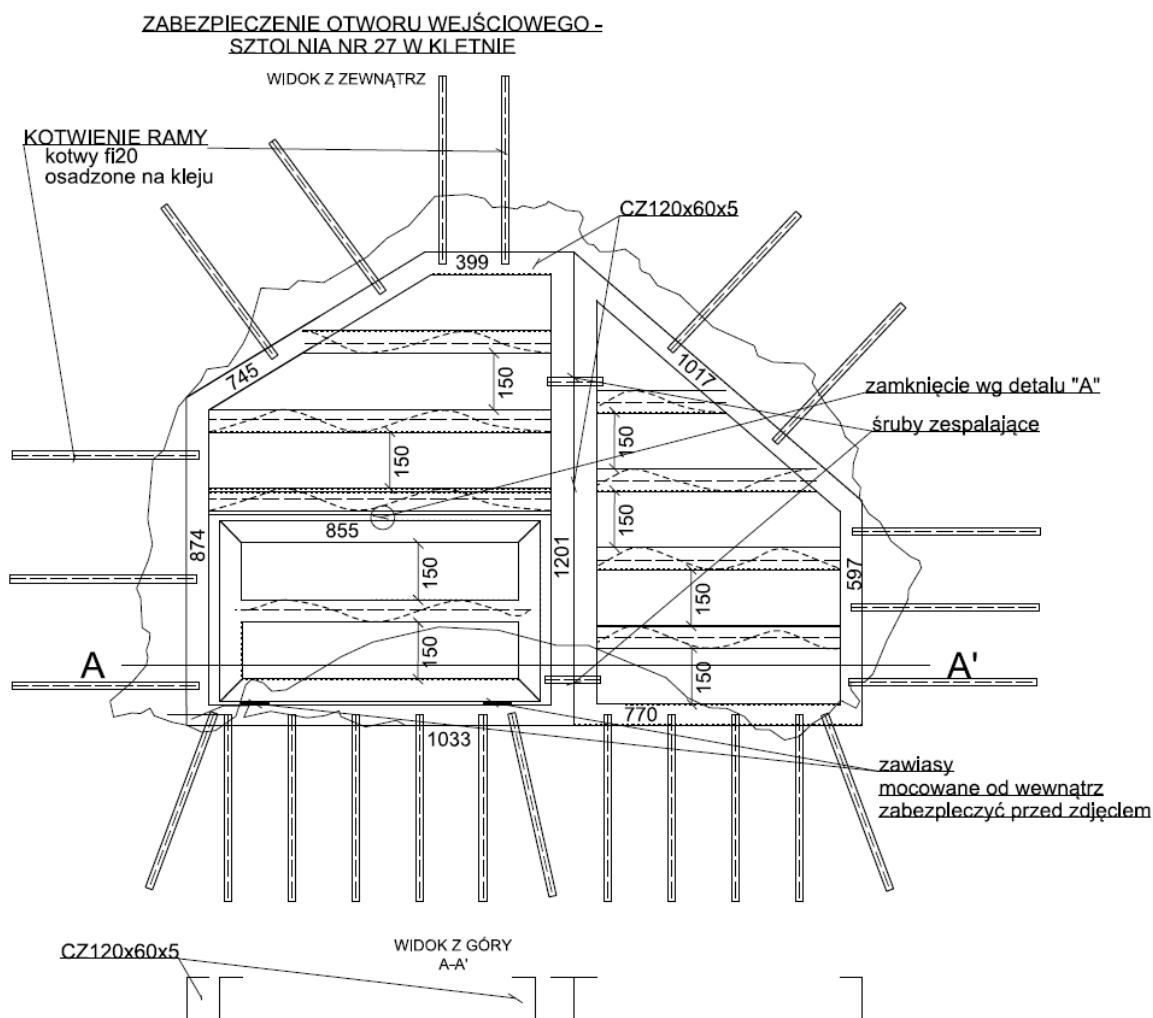
Rys. 7. Orientacyjny szkic wykonania i montażu kraty zabezpieczającej wlot do sztolni nr 27 w Kletnie.
