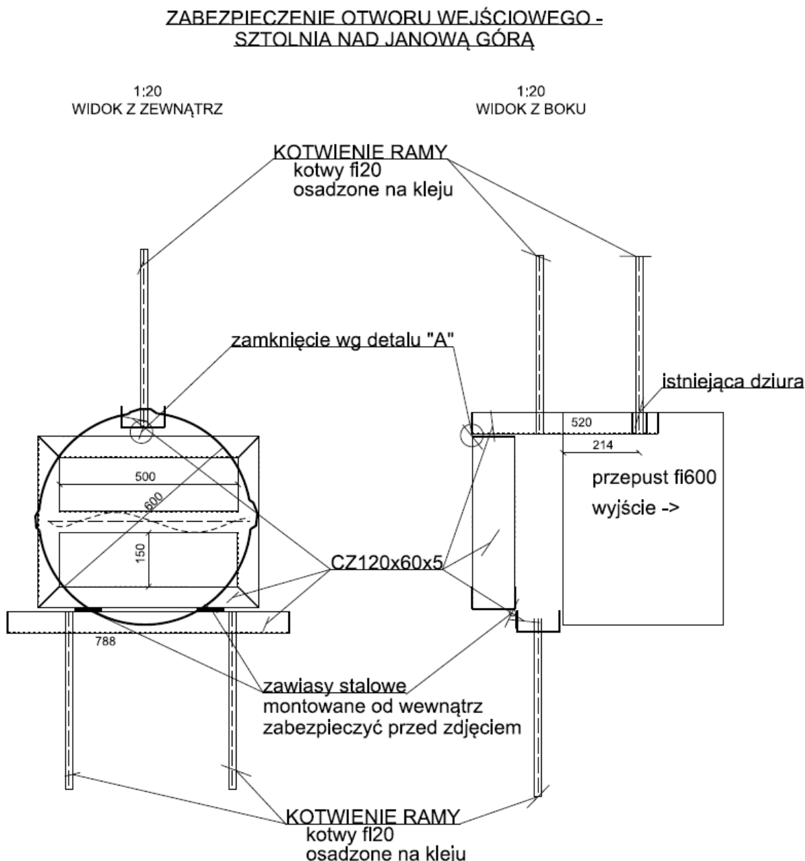
Ryc. 9. Szkic poglądowy projektu kraty zabezpieczającej wlot do sztolni nad Janową Górą.
