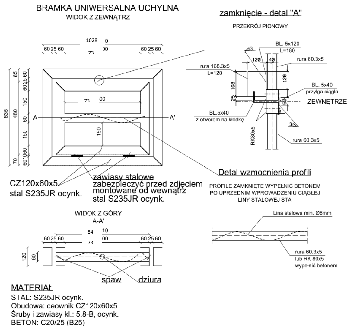
Ryc. 2. Szczegóły techniczne wykonania bramki wejściowej w sztolni nr 17 w Kletnie.
