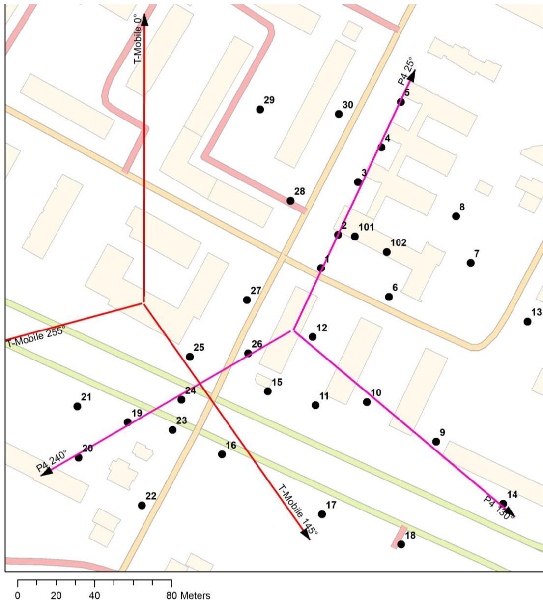
Rys. 1: Plan terenu, na którym znajduje się badana stacja bazowa
