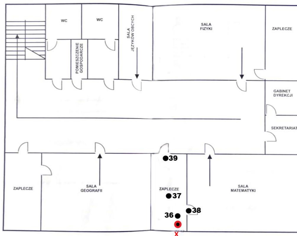
Rys. 1d: Plan rozmięszczenia punktów pomiarowych – I piętro (nowe skrzydło), kolorem czerwonym oznaczono lokalizację punktów dostępowych
