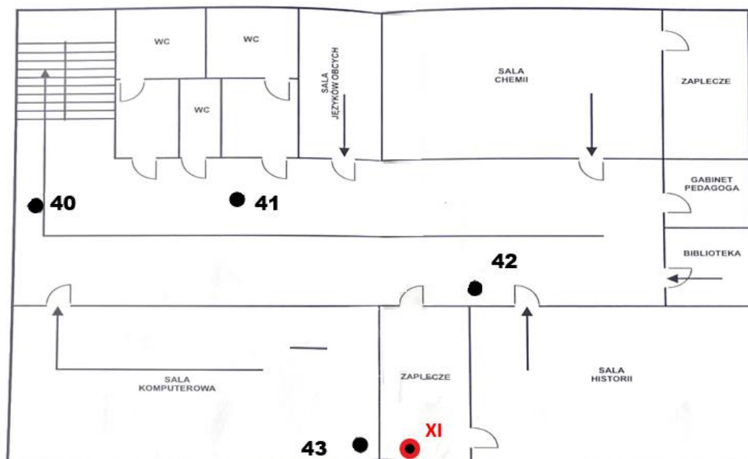
Rys. 1e: Plan rozmieszczenia punktów pomiarowych – 2 piętro (nowe skrzydło), kolorem czerwonym oznaczono lokalizację punktów dostępowych
