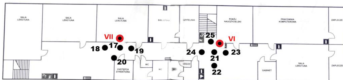
Rys. 1b: Plan rozmieszczenia punktów pomiarowych – I piętro (stare skrzydło), kolorem czerwonym oznaczono lokalizację punktów dostępowych
