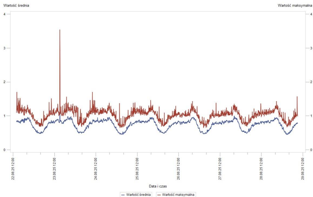
Rys. 7 Wyniki pomiarów – Budynek usługowy, Tarnowskie Góry w dniach 22.08.2025 r. – 29.08.2025 r. – wartość średnia i wartość maksymalna
