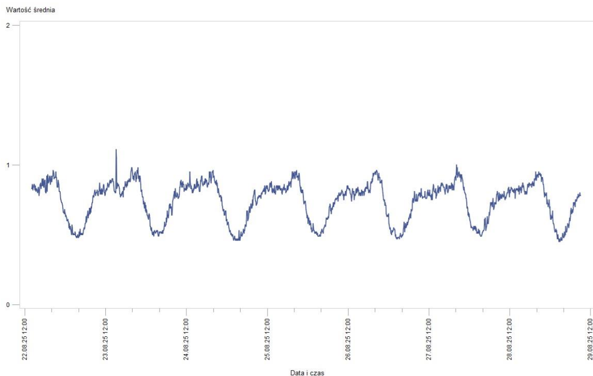
Rys. 6 Wyniki pomiarów – Budynek usługowy, Tarnowskie Góry w dniach 22.08.2025 r. – 29.08.2025 r. – wartość średnia
