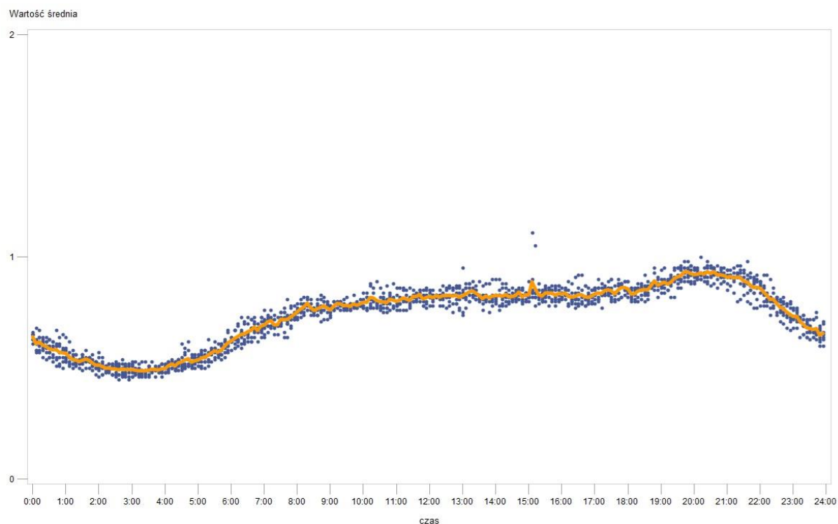
Rys. 8 Wyniki pomiarów – Budynek usługowy, Tarnowskie Góry – średnia za okres 24 godzin
