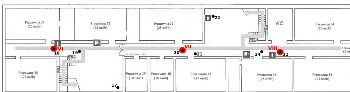
Rys. 1c: Plan rozmieszczenia punktów pomiarowych – I piętro, kolorem czerwonym oznaczono lokalizację punktów dostępowych
