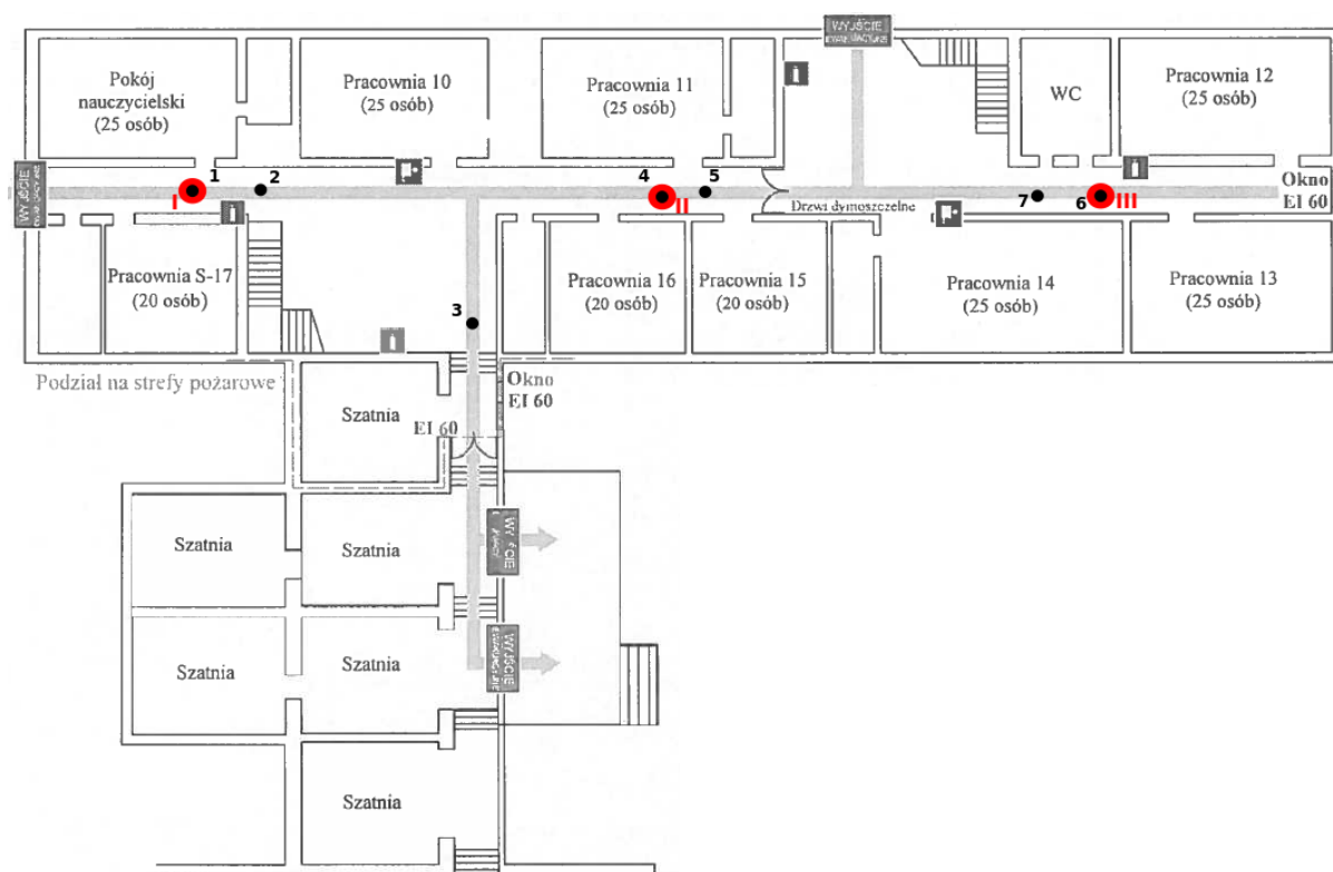
Rys. 1b: Plan rozmieszczenia punktów pomiarowych – parter, kolorem czerwonym oznaczono lokalizację punktów dostępnych
