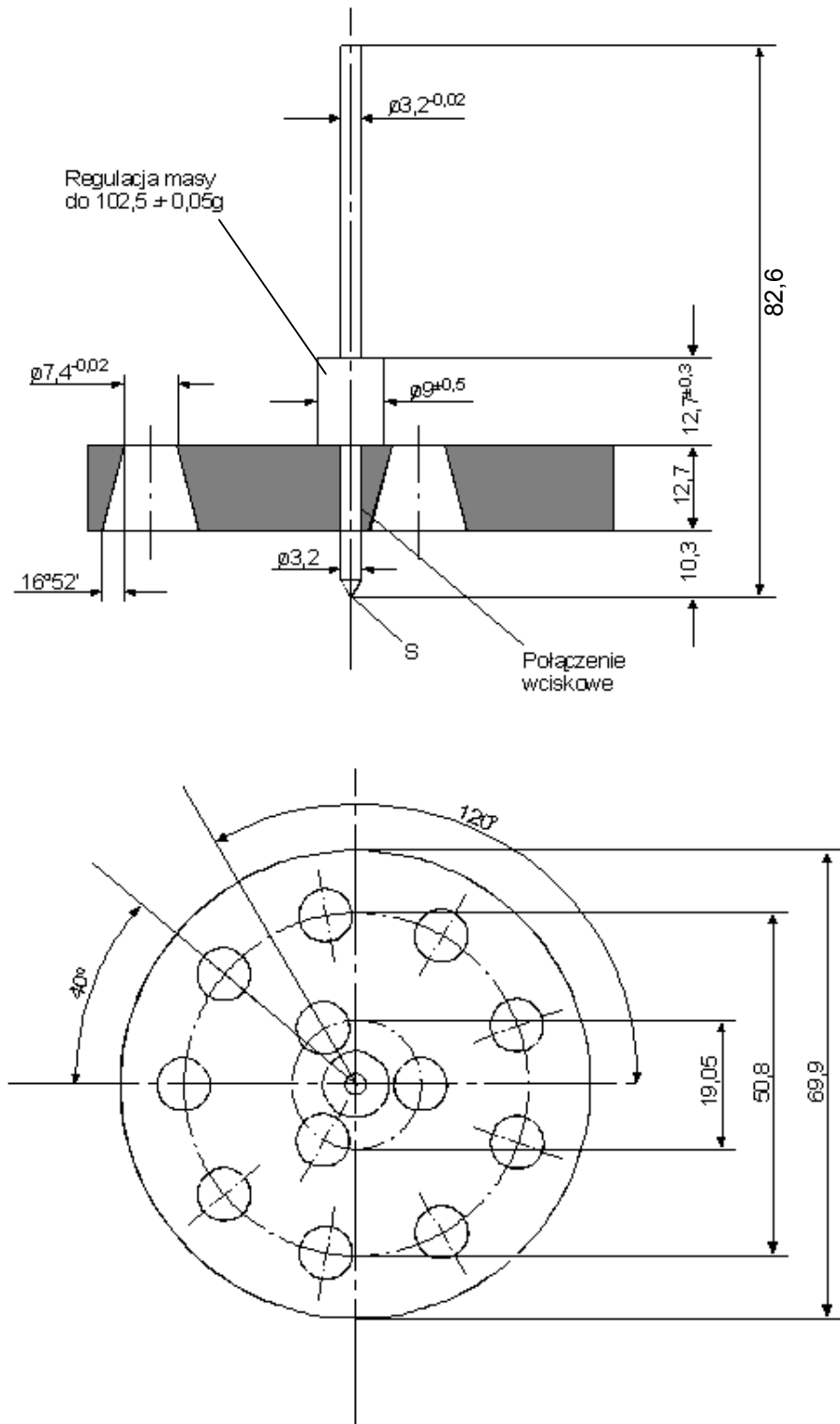
Rysunek 1. Penetrometr
