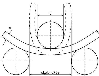
Schemat próby na zginanie
